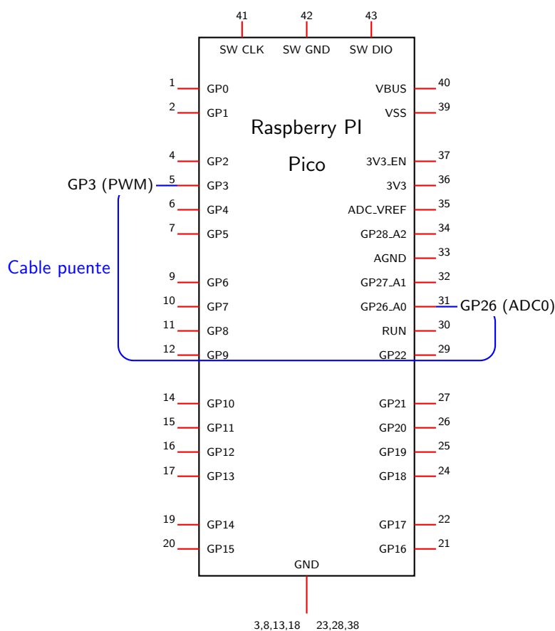
Figura 5: Conexión física: cable puente entre GP3 (salida PWM) y GP26 (entrada ADC) en la Raspberry Pi Pico 2W.
