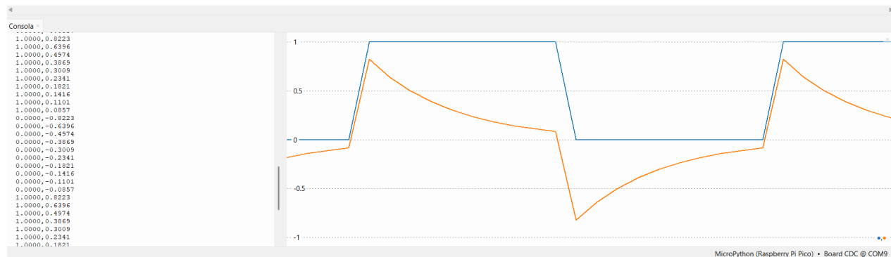
Figura 8: Filtro pasa altas a f = 50 Hz.
