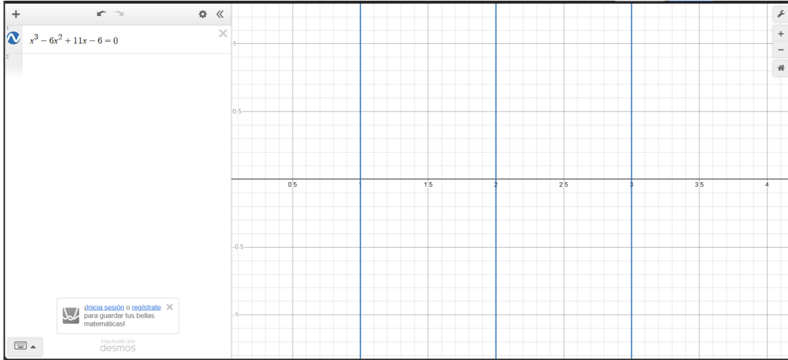
Figura 4: Se nos muestra la gráfica de la ecuación x^3 - 6x^2 + 11x - 6 = 0 con esto, de igual forma se observan las raíces reales en x = 1 , x = 2 y x = 3 .
