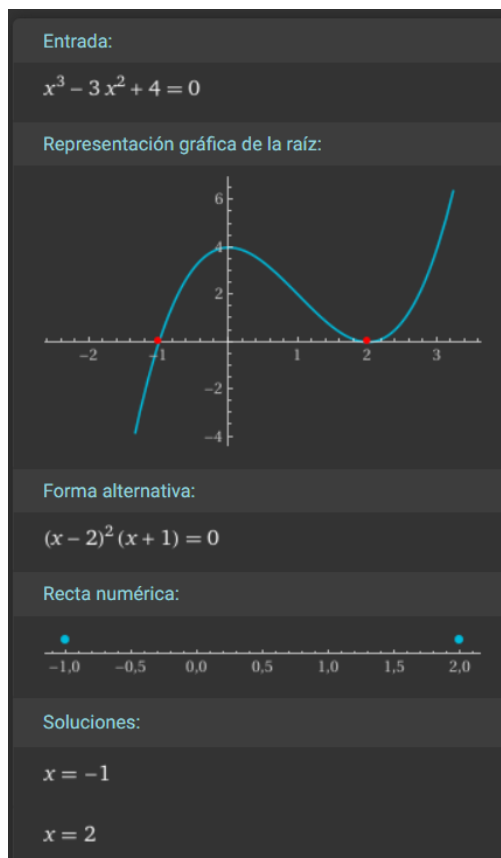
Figura 10: Comprobación matemática de la función cúbica en Wolfram Alpha.
