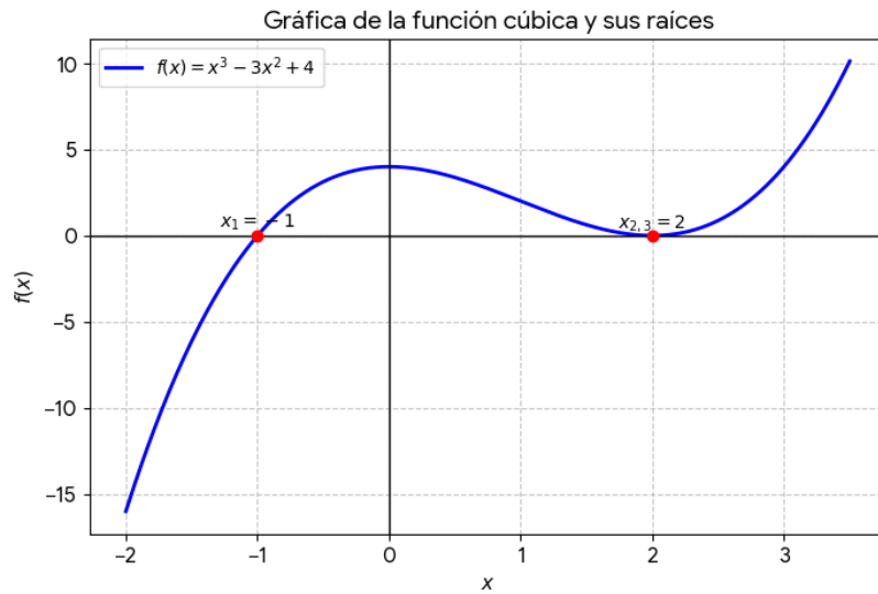
Figura 9: Gráfica de la función cúbica señalando la raíz repetida.
