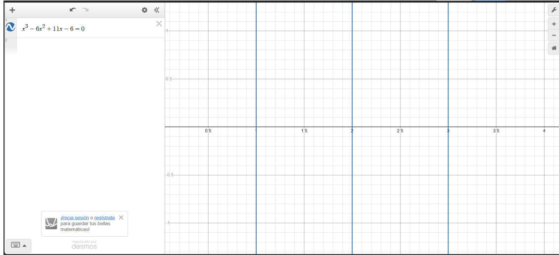
Figura 7: Se nos muestra la gráfica de la ecuación x^3 - 6x^2 + 11x - 6 = 0 con esto, de igual forma se observan las raíces reales en x = 1 , x = 2 y x = 3 .
