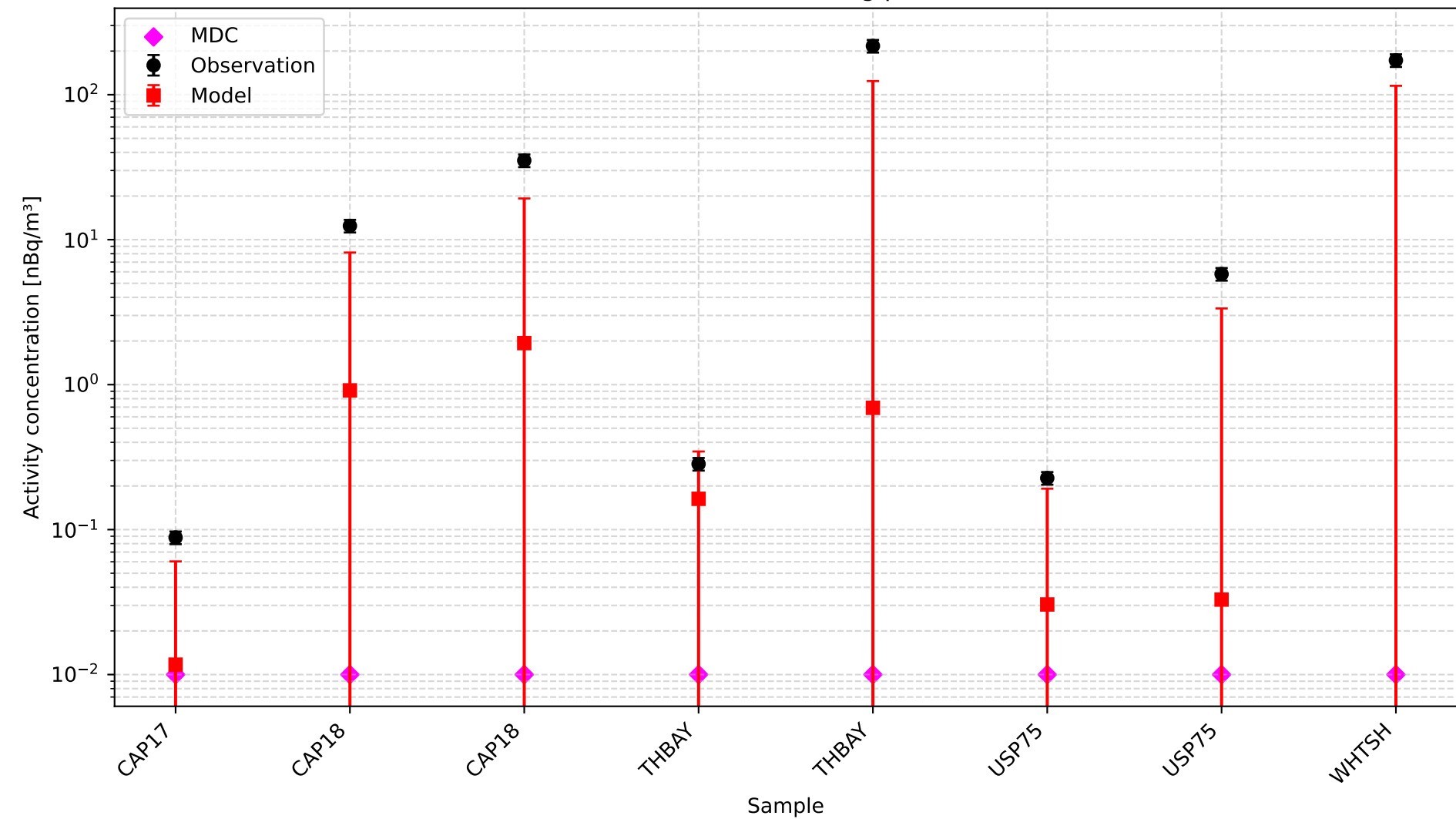
Modelled concentrations using posterior mode
