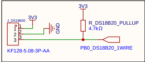
Sensor DS18B20 Temp
