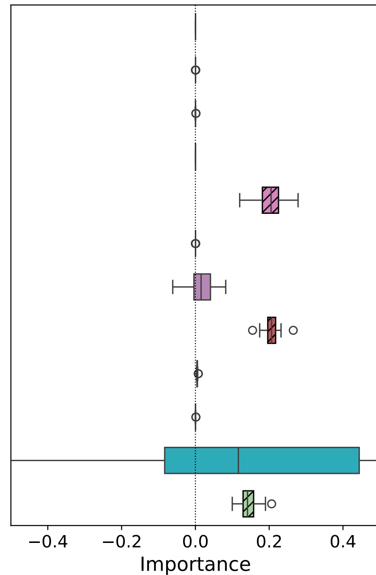
SVR R^2 = 0.77
