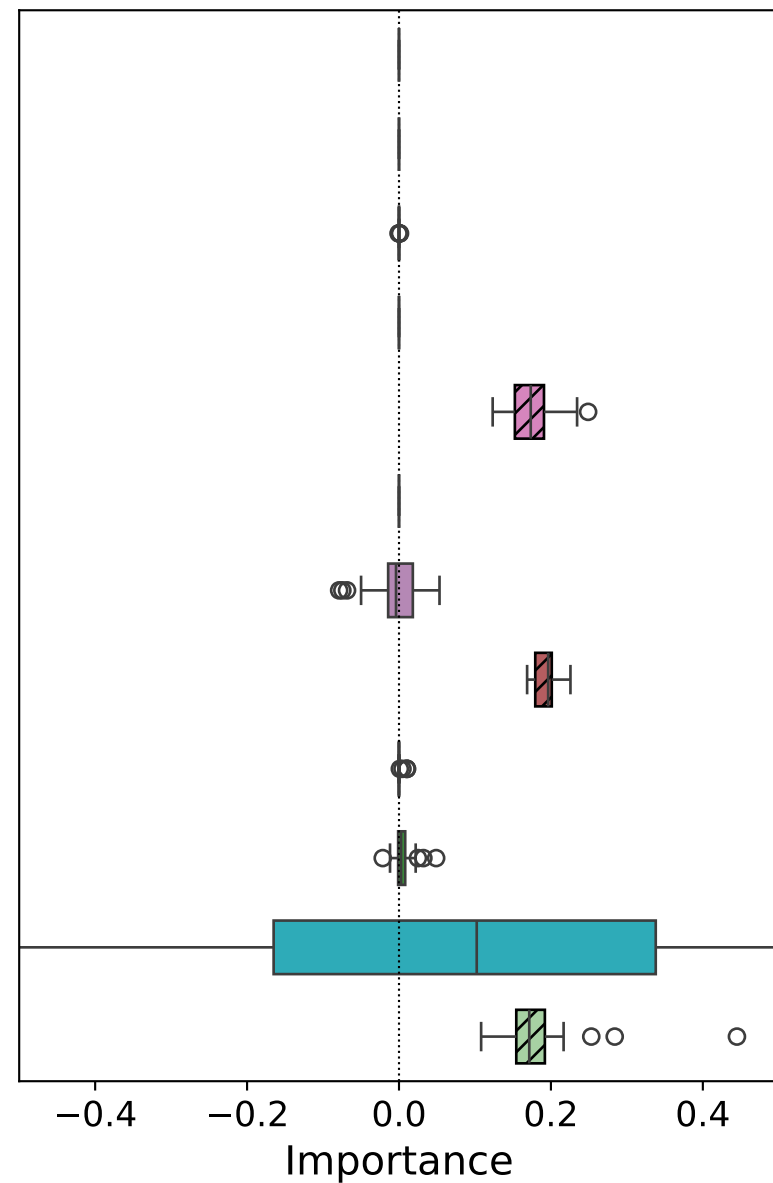
GB R^2 = 0.89
