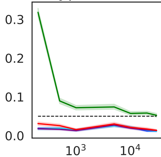
Type-I error
