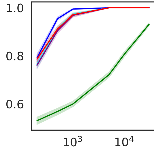
AUC
