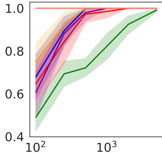
AUC
