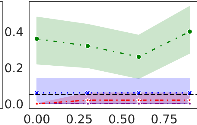
Type-I Error
