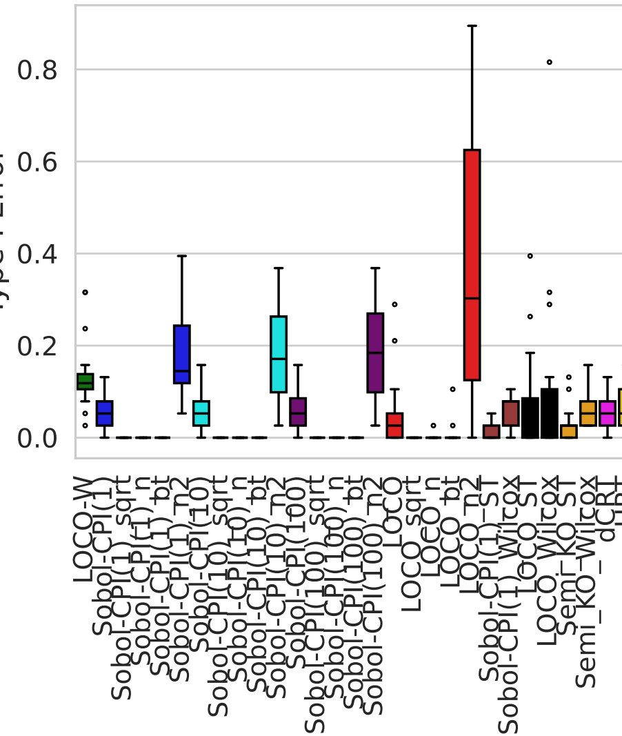
Type-I Error
