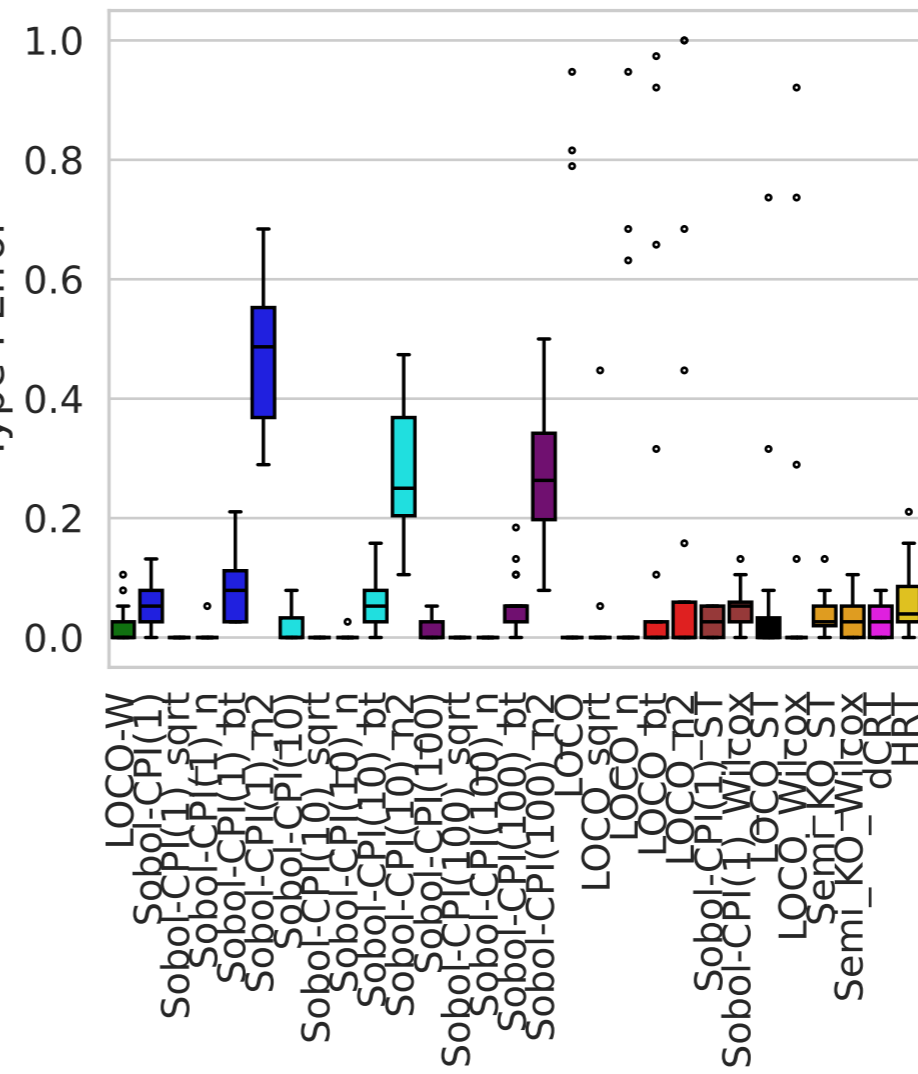
Type-I Error
