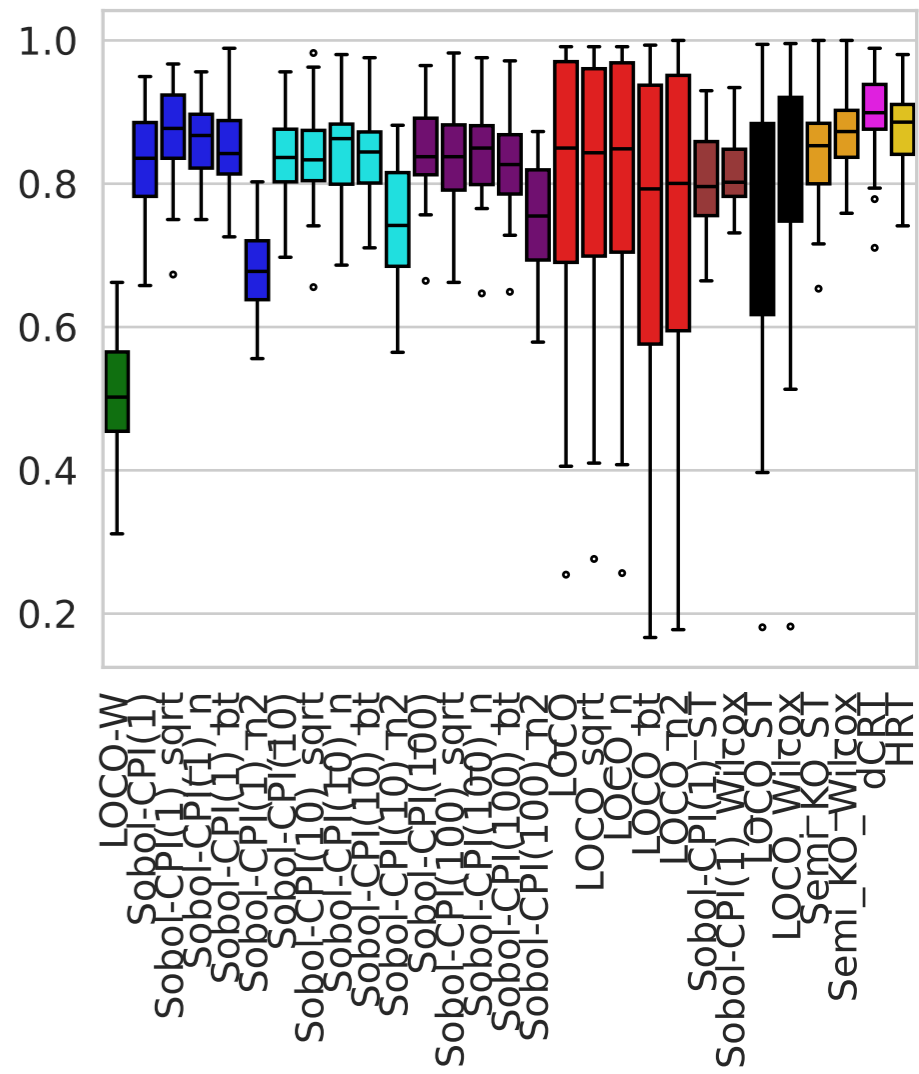
AUC
