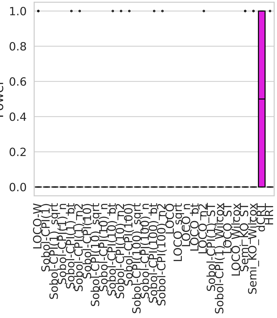
Type-I Error
