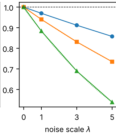
GHZ, 6 qubits
