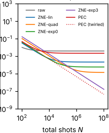
untwirled, d=5
