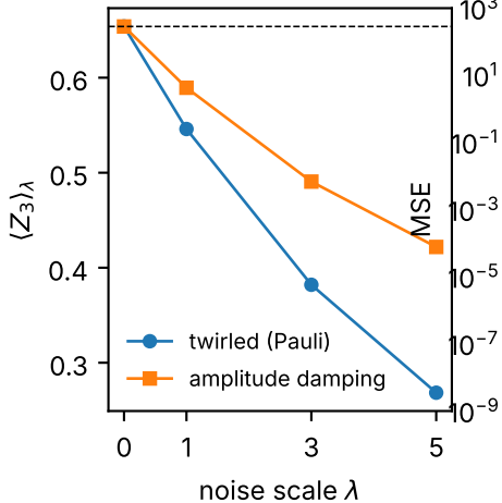
TFIM d=5
