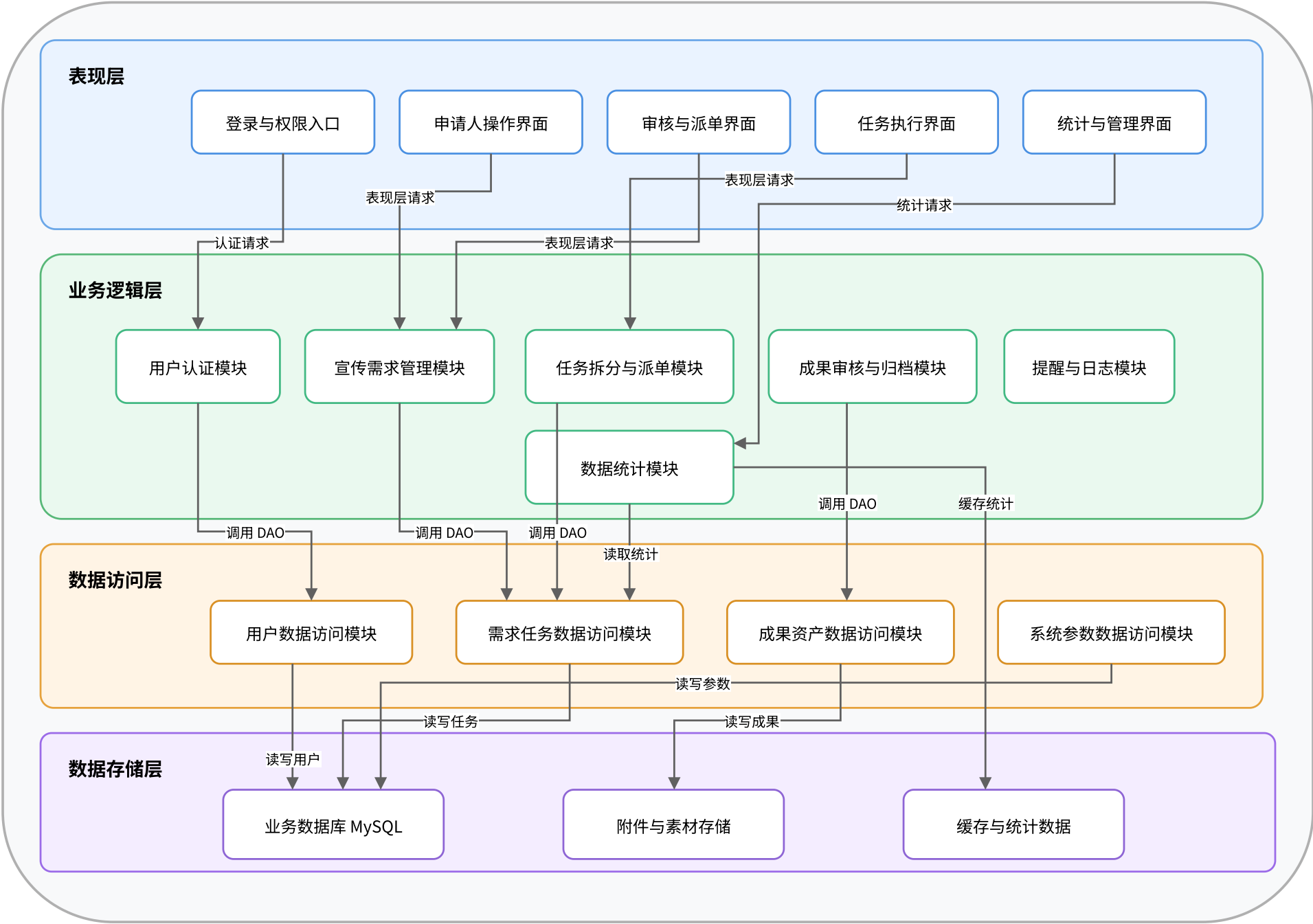
学院宣传工作智能协同管理平台总体架构图
