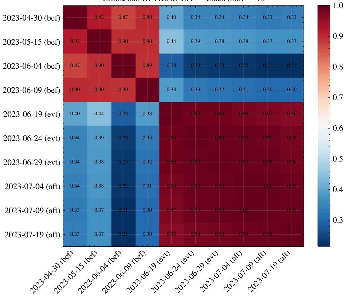
Cosine sim OPTICAL TxT — token (3,6) — v3
