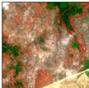
fid 25 · tile_0 · 2023-10-12 · evt Fire scar
