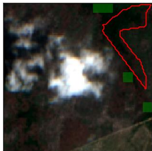
fid 25 · tile_0 · 2023-11-11 · aft Fire scar
