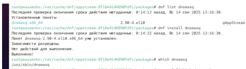
Рис. 2.17: Установка пакетов
