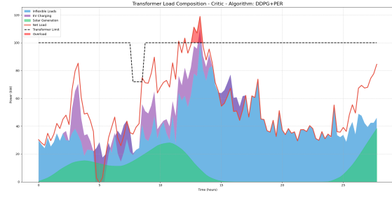
(b) DDPG+PER
