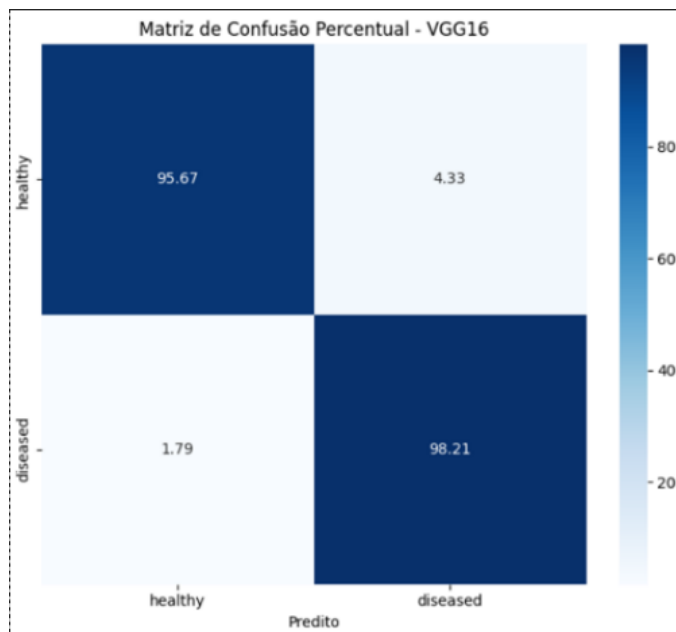
Fig. 4. Matriz de Confusão para o Modelo VGG16, Fonte: Autoria própria (2025).
