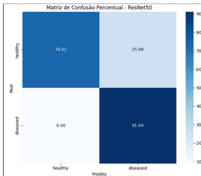
Fig. 3. Matriz de Confusão para o Modelo ResNet50, Autoria própria (2025).
