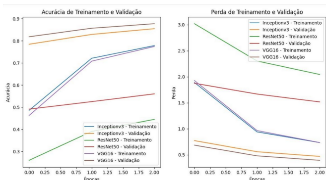
Fig. 1. Curvas de Acurácia e Perda para o Modelo InceptionV3, ResNet50 e VGG16, Fonte: Autoria própria (2025).
