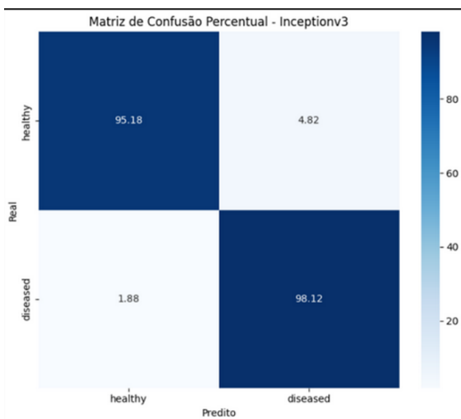
Fig. 2. Matriz de Confusão para o Modelo InceptionV3, Fonte: Autoria própria (2025).
