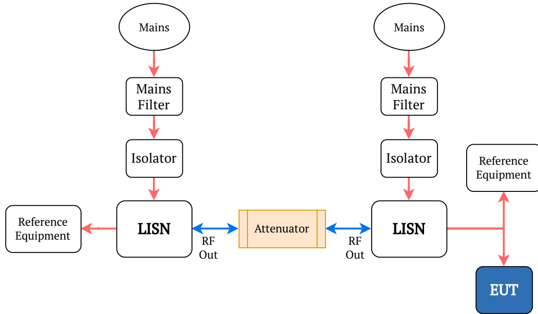
Figura 5.1: Esquema del montaje del estudio de sensibilidad PLC: dos LISN con sus salidas de RF interconectadas a través de un atenuador variable, con la PL460-EK remota en el lado A y el EUT junto a la PL460-EK de referencia en el lado B.
