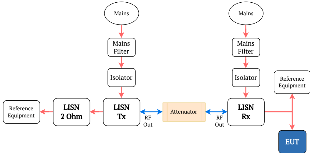
Figura 5.1: Esquema del montaje del estudio de sensibilidad PLC: dos LISN con sus salidas de RF interconectadas a través de un atenuador variable, con la PL460-EK remota en el lado A y el EUT junto a la PL460-EK de referencia en el lado B.
