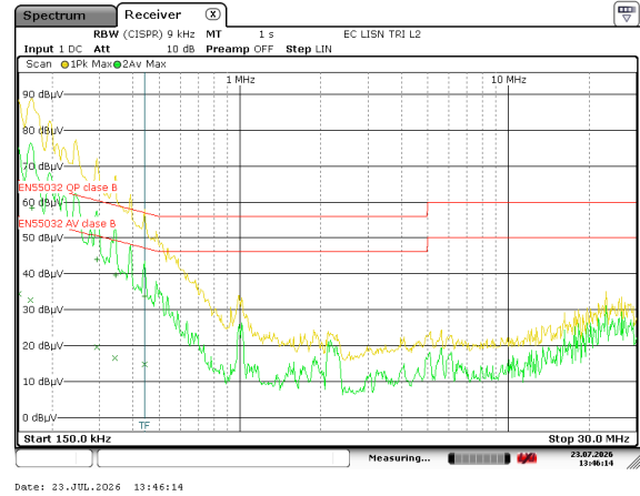
(b) Fase L2 ( S ).
