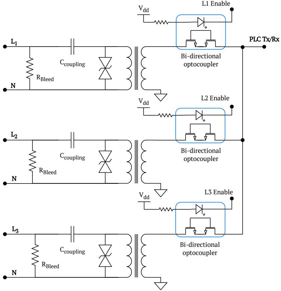
Figura 3.3: Diagrama de acoplamiento trifásico pasivo con selección de fase.
