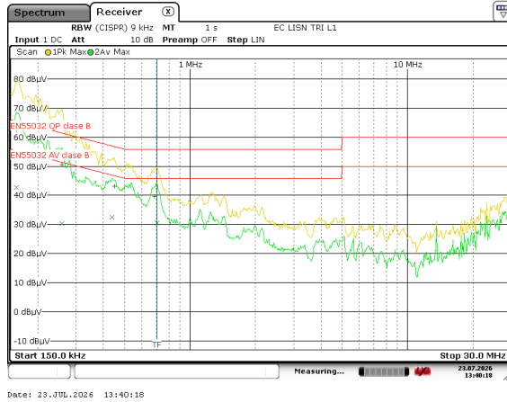
(a) Fase L1 ( R ).
