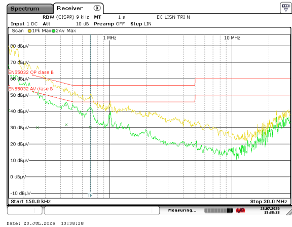
(d) Neutro ( N ).
