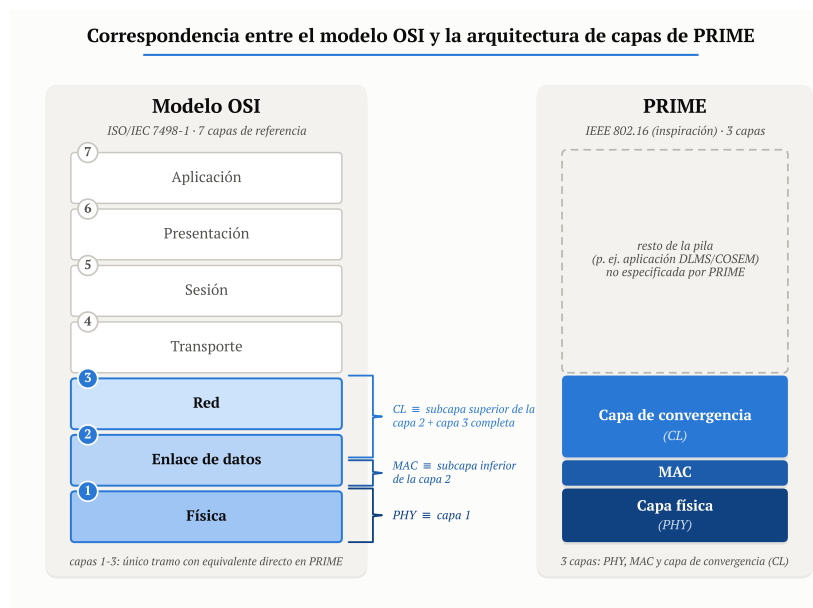
Figura 2.5: Comparativa simplificada entre el modelo de referencia OSI y la arquitectura de capas del protocolo PRIME (PHY, MAC y capa de convergencia).
