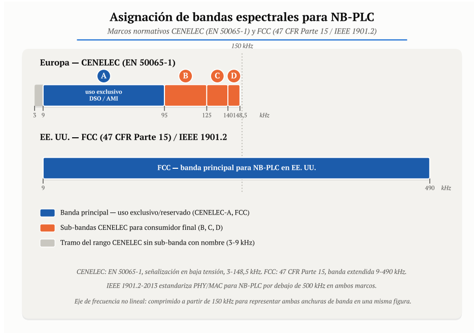
Figura 2.7: Asignación de bandas espectrales para NB-PLC según los estándares CENELEC y FCC.
