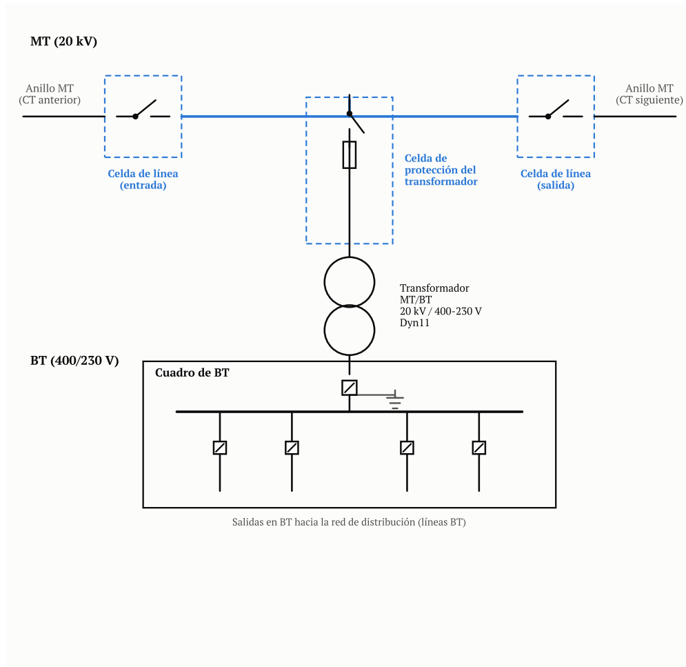
Figura 2.4: Esquema unifilar simplificado de un centro de transformación MT/BT, con celdas de línea de entrada/salida en anillo, celda de protección del transformador y cuadro de baja tensión.
