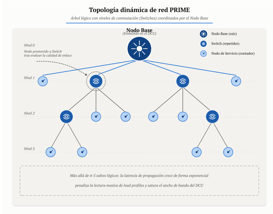
Figura 2.6: Topología dinámica de red PRIME con niveles de conmutación ( Switches ) coordinados por el Nodo Base.
