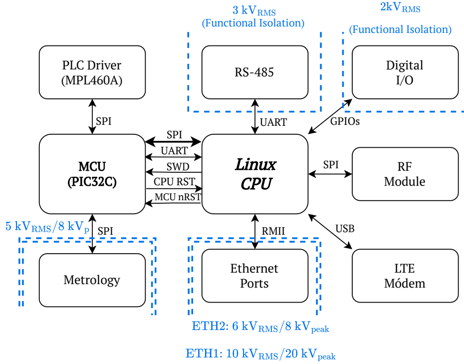
Figura 3.2: Diagrama de interconexión entre bloques y periféricos del sistema.
