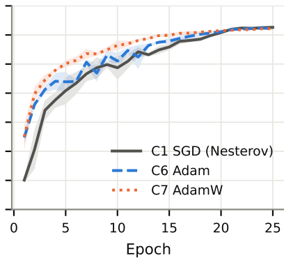
Optimiser
