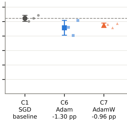
Optimiser
