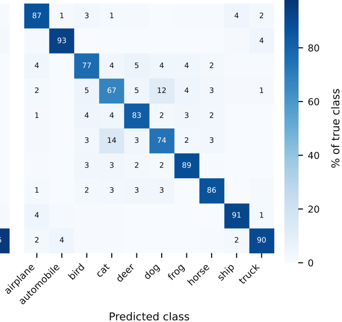
C2 Simple CNN (worst)
