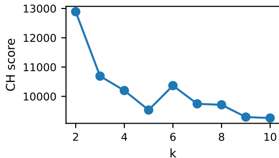
Calinski-Harabasz
