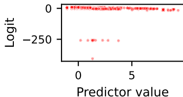
flow_iat.min
