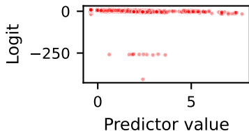
fwd_iat.min
