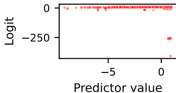
id.orig_p
