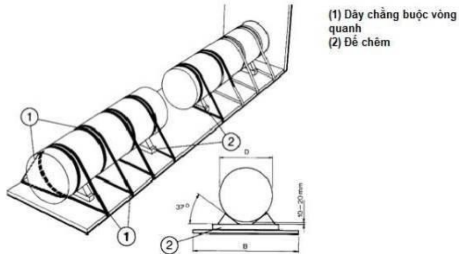
Hình 4.7. Minh họa mô tả về vận chuyển dầm tròn cho công trình xây dựng
