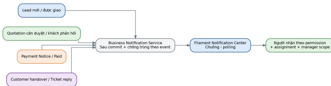
Hình 5. Cơ chế thông báo nghiệp vụ
