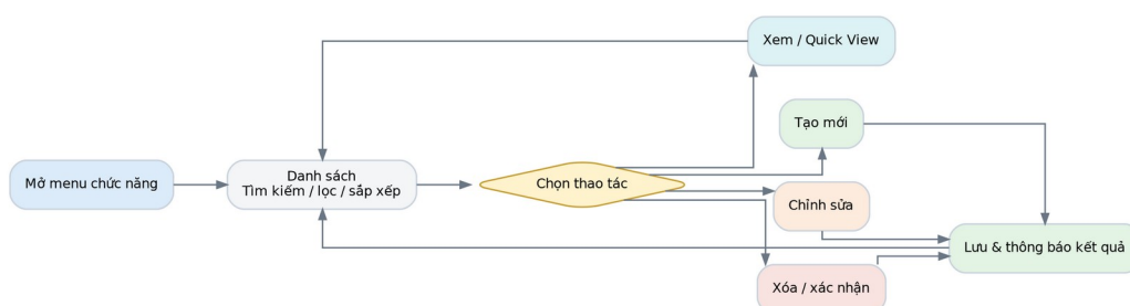
Sơ đồ activity/visual áp dụng cho Segments
