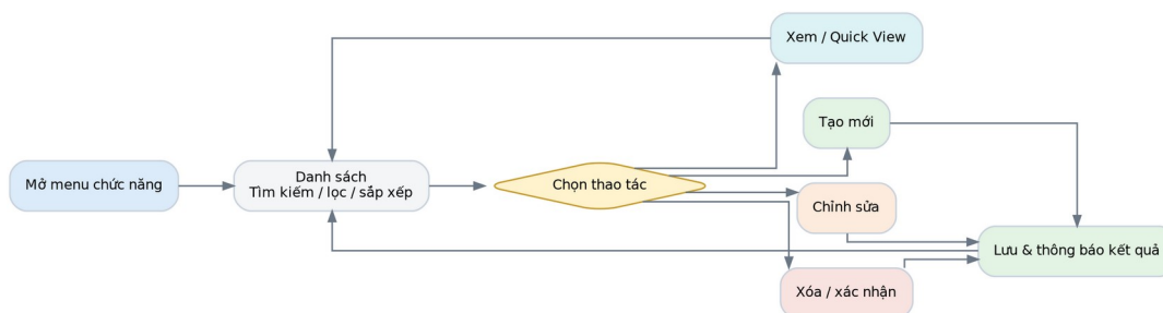
Hình 4. Quy trình chuẩn khi làm việc với một màn hình dữ liệu
