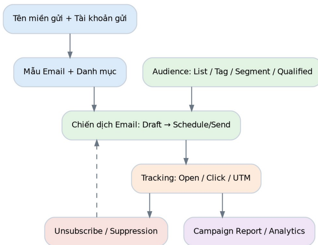
Sơ đồ tổng quan: Email
