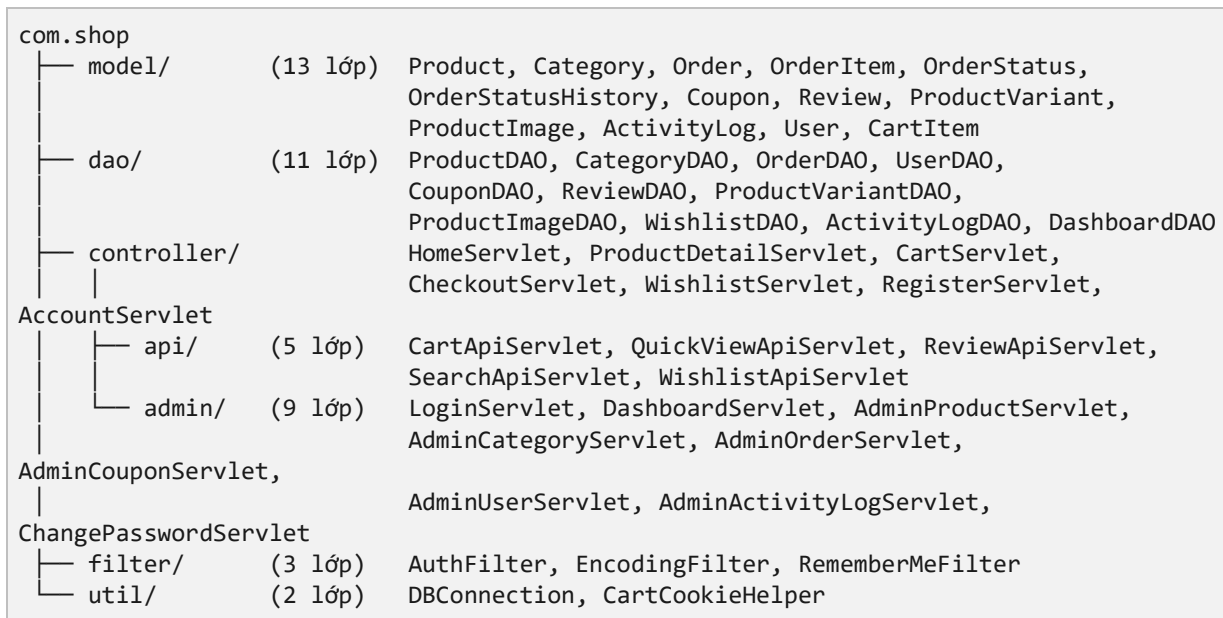
Hình 3.3: Sơ đồ tổ chức package mã nguồn (khoảng 50 lớp Java)
