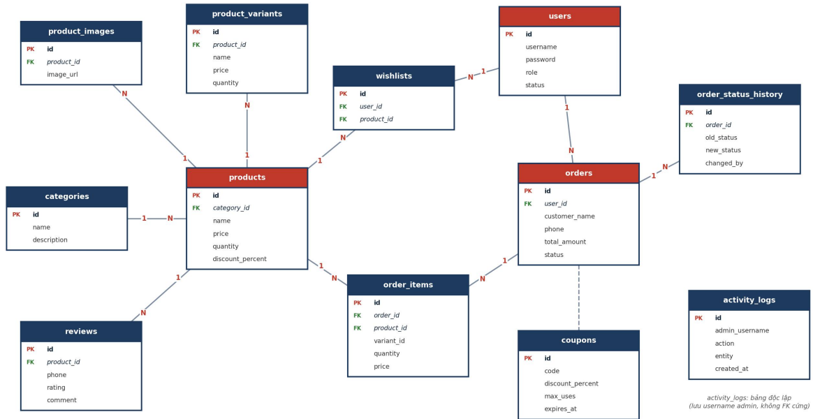
Hình 4.1: Sơ đồ quan hệ thực thể (ERD) của cơ sở dữ liệu shop_db
