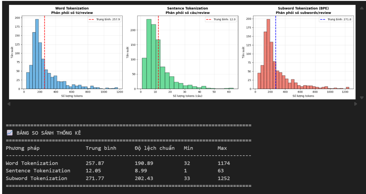
Hình 27: Phân phối và bảng so sánh thống kê giữa các phương pháp Tokenization
