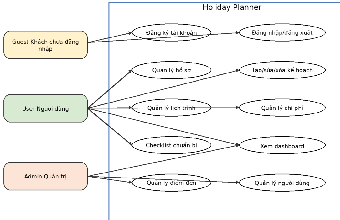
Hình 2.2. Sơ đồ Use Case tổng thể
