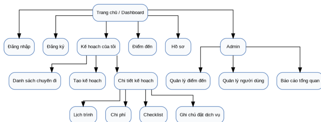
Hình 2.5. Site map dự kiến của hệ thống
