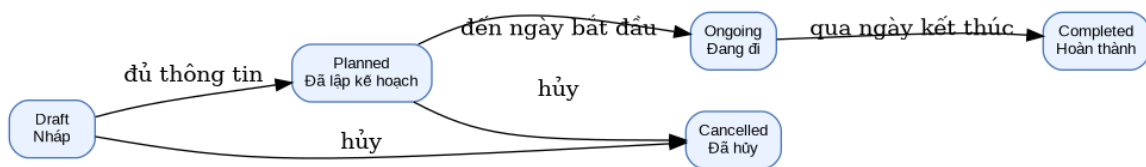
Hình 2.4. Sơ đồ chuyển trạng thái kế hoạch chuyến đi
