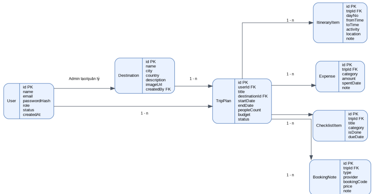
Hình 2.1. Sơ đồ quan hệ đối tượng của hệ thống Holiday Planner
