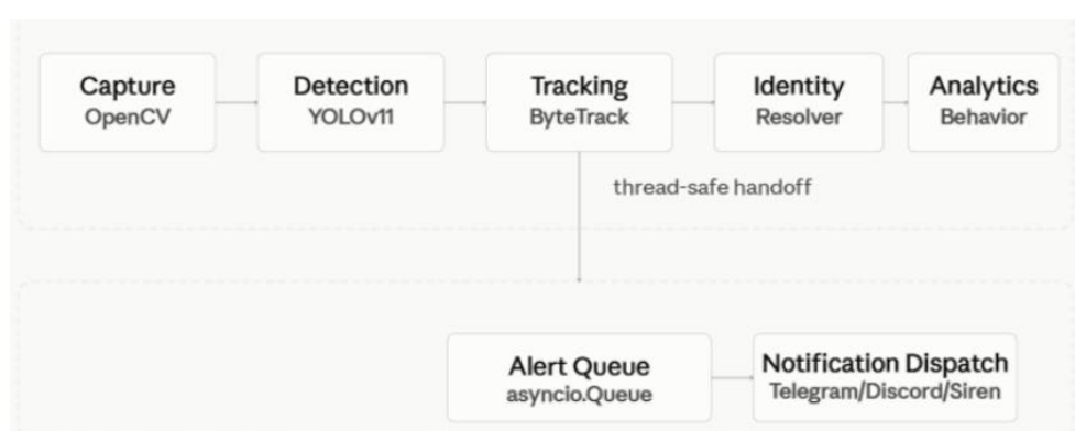
Hình 20: Kiến trúc pipeline sáu tầng của hệ thống
