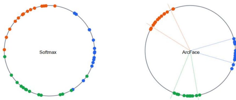
Hình 8: So sánh không gian đặc trưng giữa Softmax truyền thống và ArcFace
