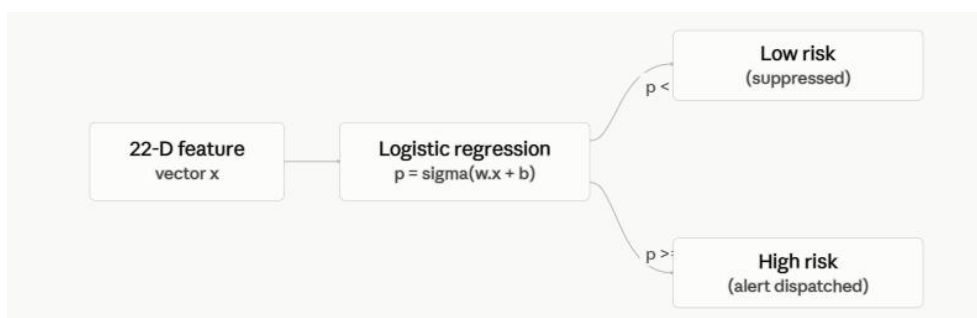
Hình 22: Sơ đồ mô hình chấm điểm rủi ro hành vi bằng hồi quy logistic
