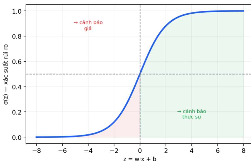
Hình 10: Hàm Sigmoid ánh xạ điểm số tuyến tính z về xác suất rủi ro trong khoảng (0,1)
