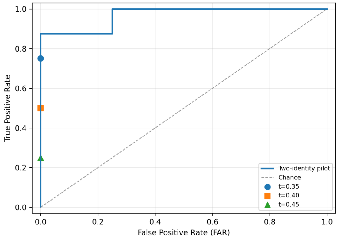
Hình 36: Đường ROC của pilot nhận diện khuôn mặt hai danh tính
