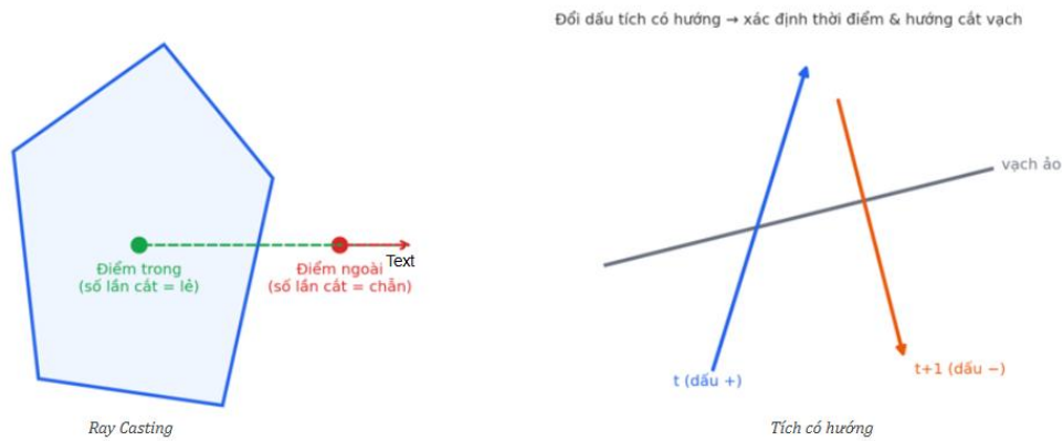
Hình 9: Hai kỹ thuật hình học tính toán dùng trong phân tích hành vi
