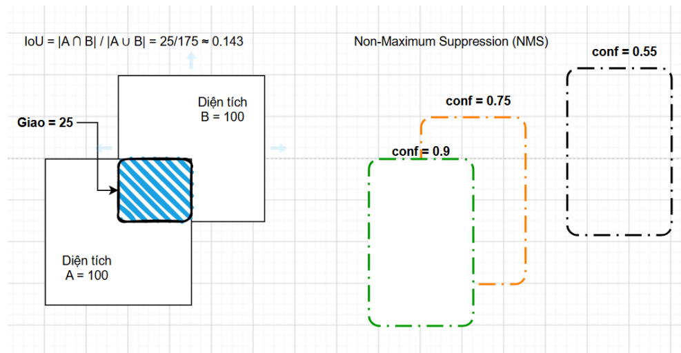
Hình 12: Minh họa IoU giữa hai khung bao và cơ chế lọc trùng lặp Non-Maximum Suppression (NMS)
