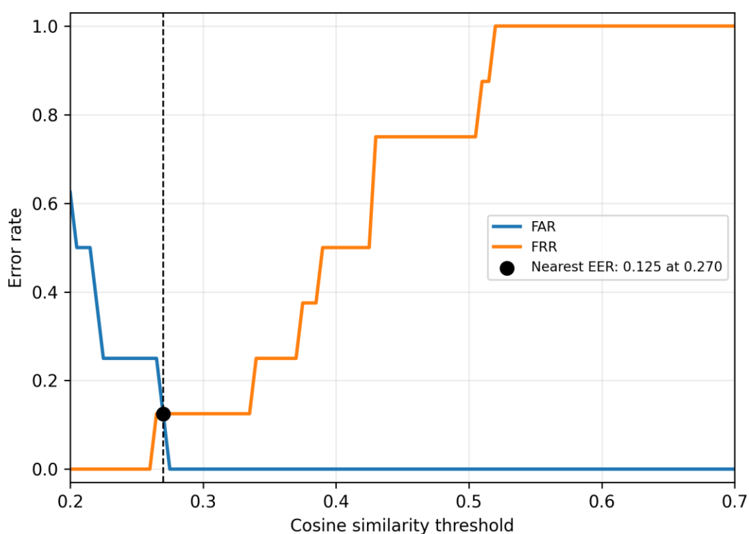
Hình 37: FAR và FRR theo ngưỡng cosine similarity trong pilot
