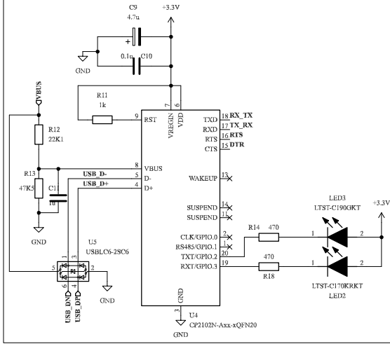
USB Module
