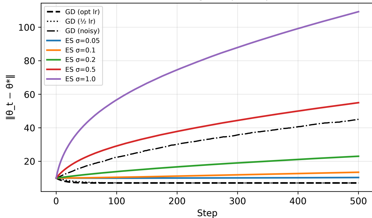
D4: Convergence per step
