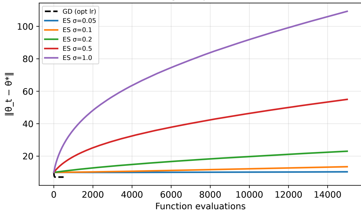
D4: Convergence per function eval
