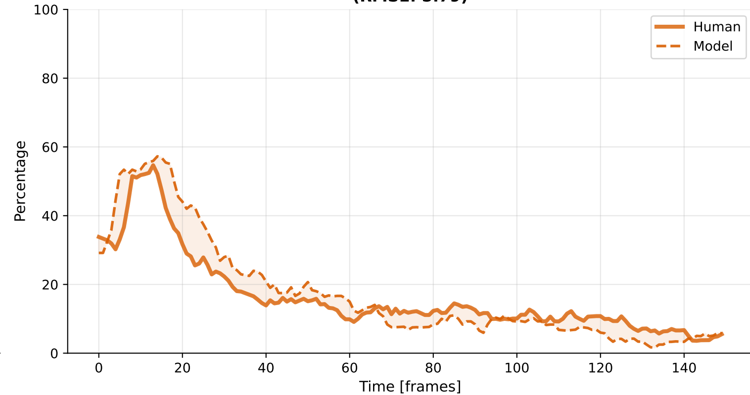
Revisit (RMSE: 3.68)
