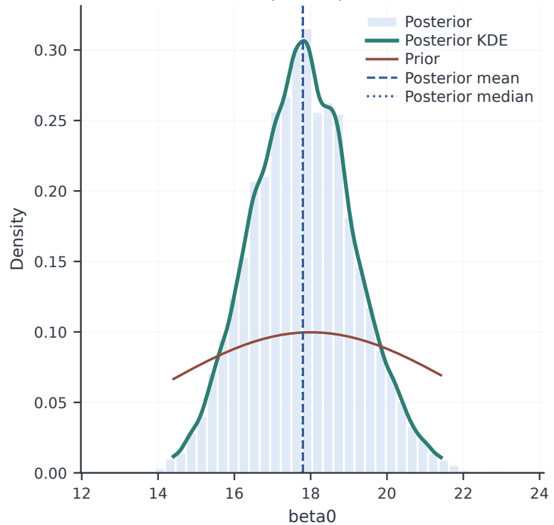
beta0: prior vs posterior
