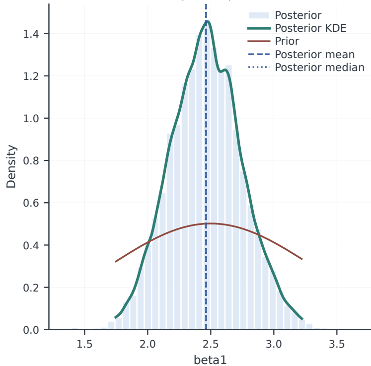
beta1: prior vs posterior
