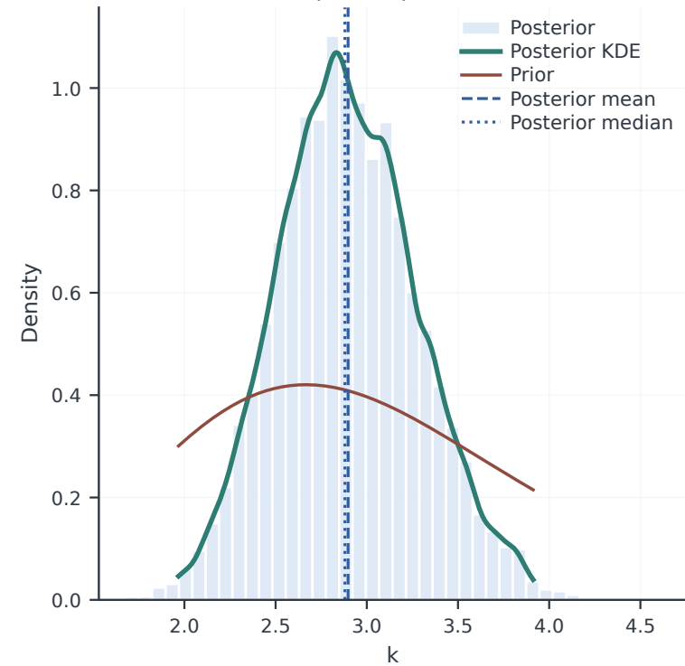
k: prior vs posterior
