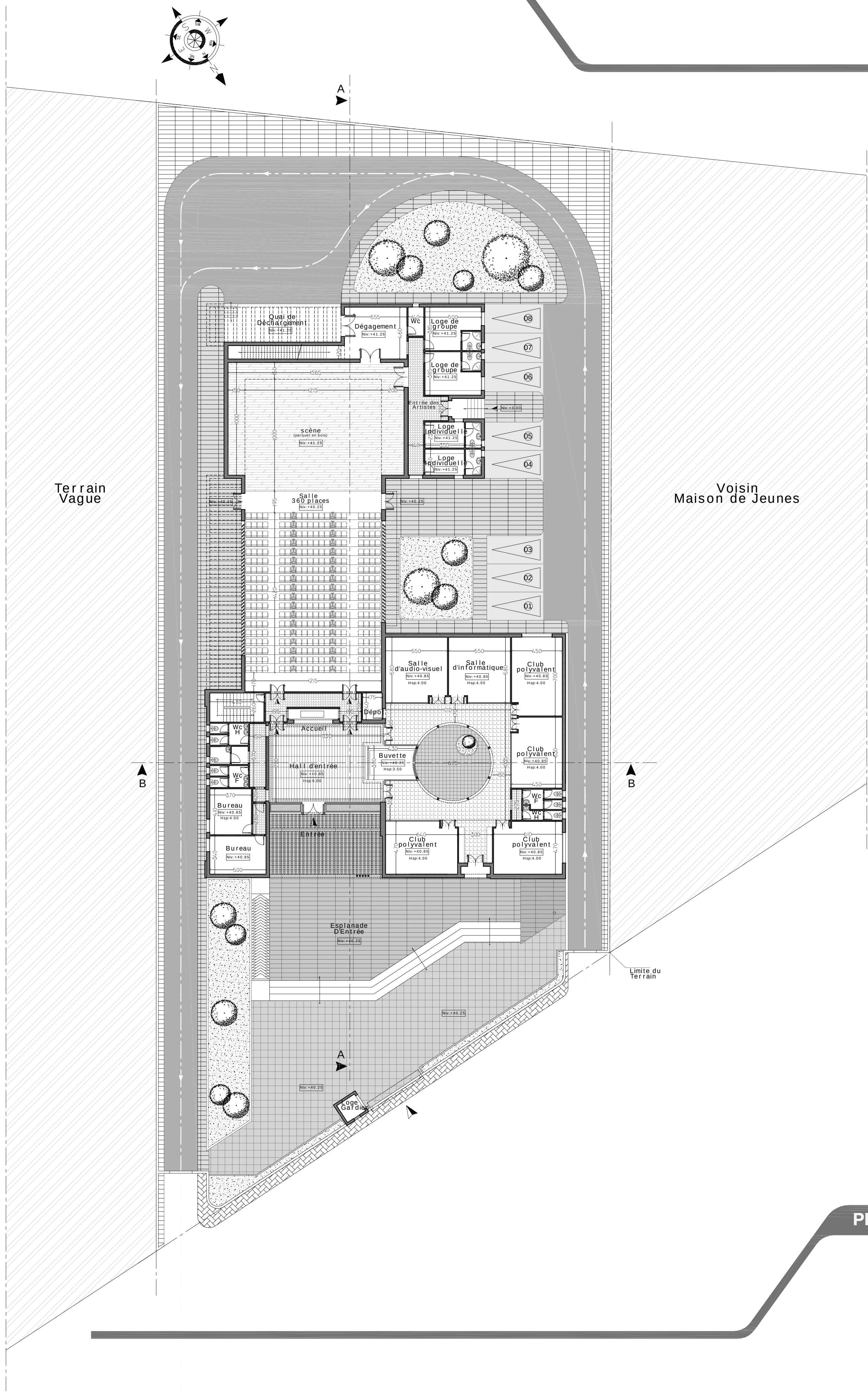
PLAN RDC ech 1/200
