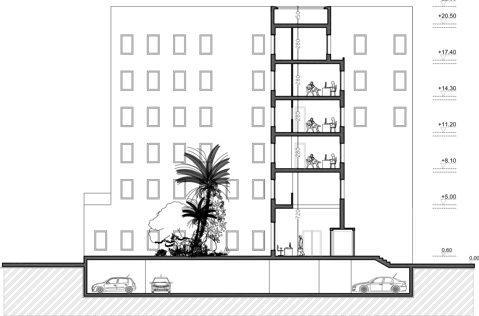
COUPE B-B
