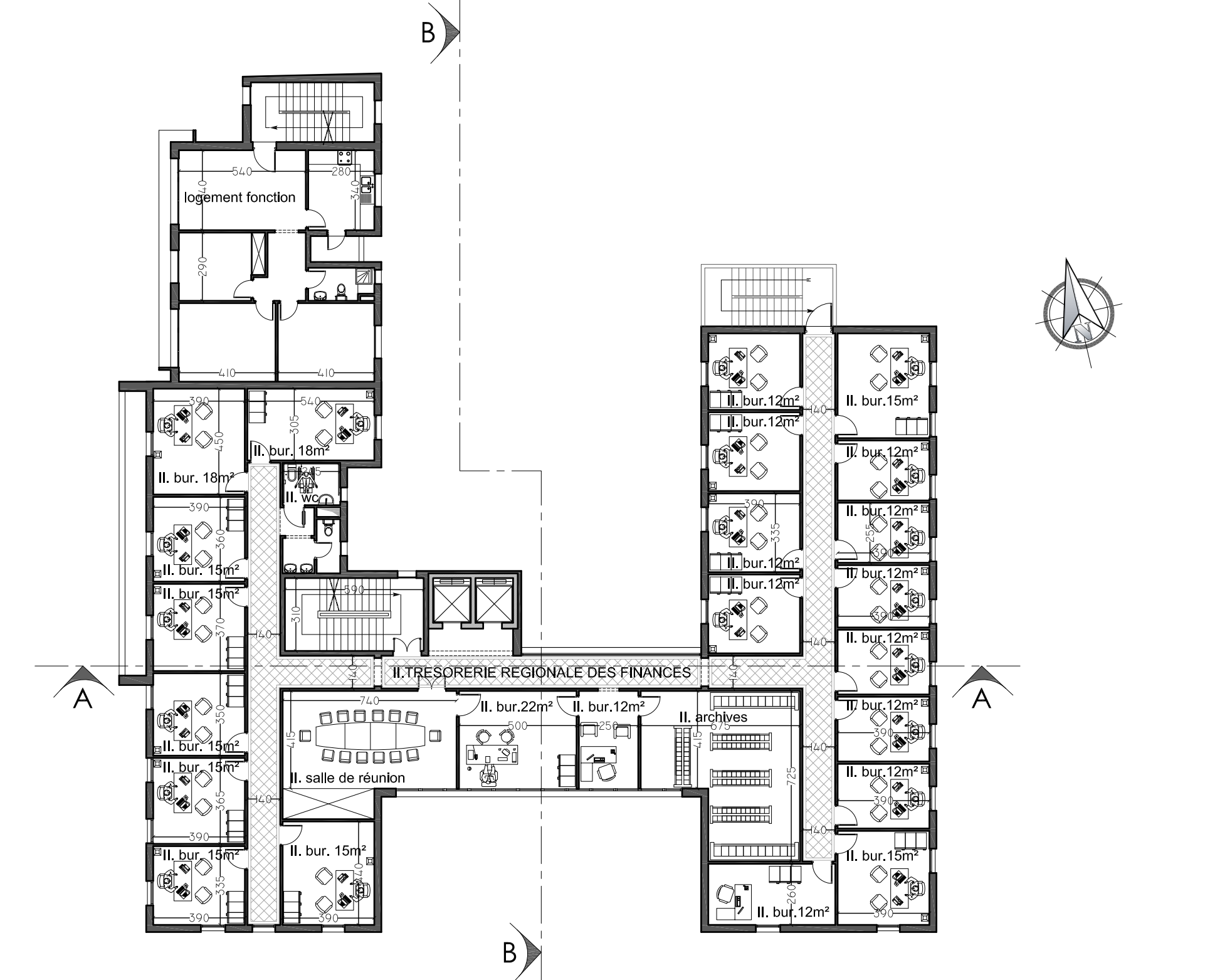
PLAN 3ème Etage ech 1/200
