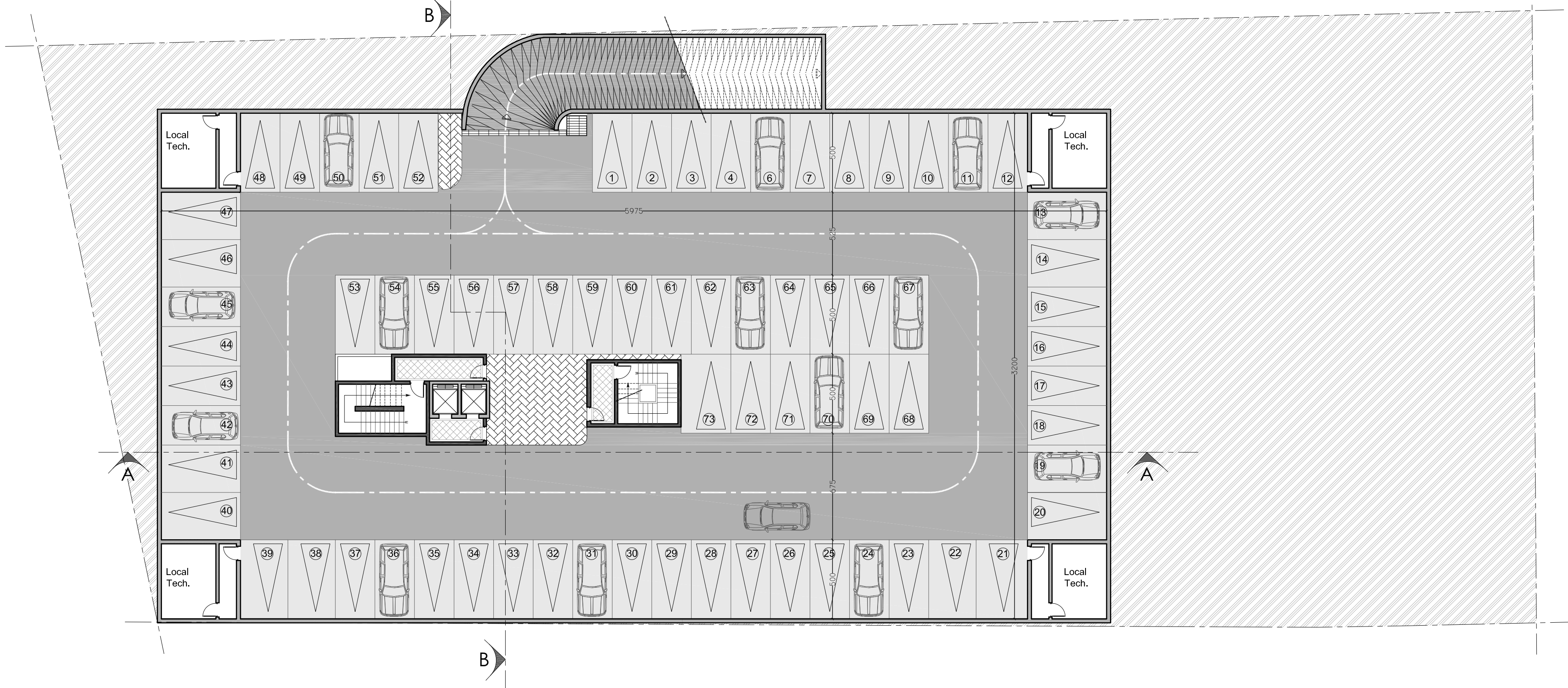
PLAN SOUS SOL ech 1/200
