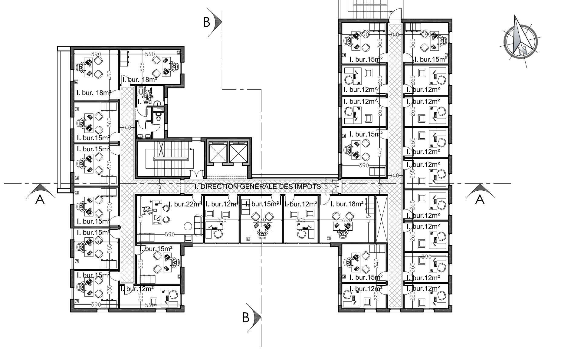
PLAN 4ème Etage ech 1/200
