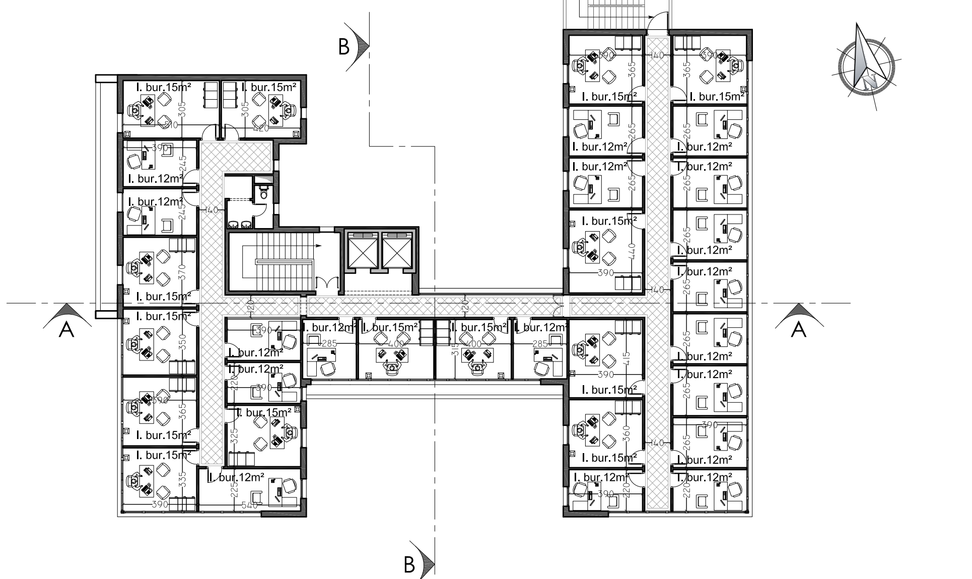
PLAN 5ème Etage ech 1/200
