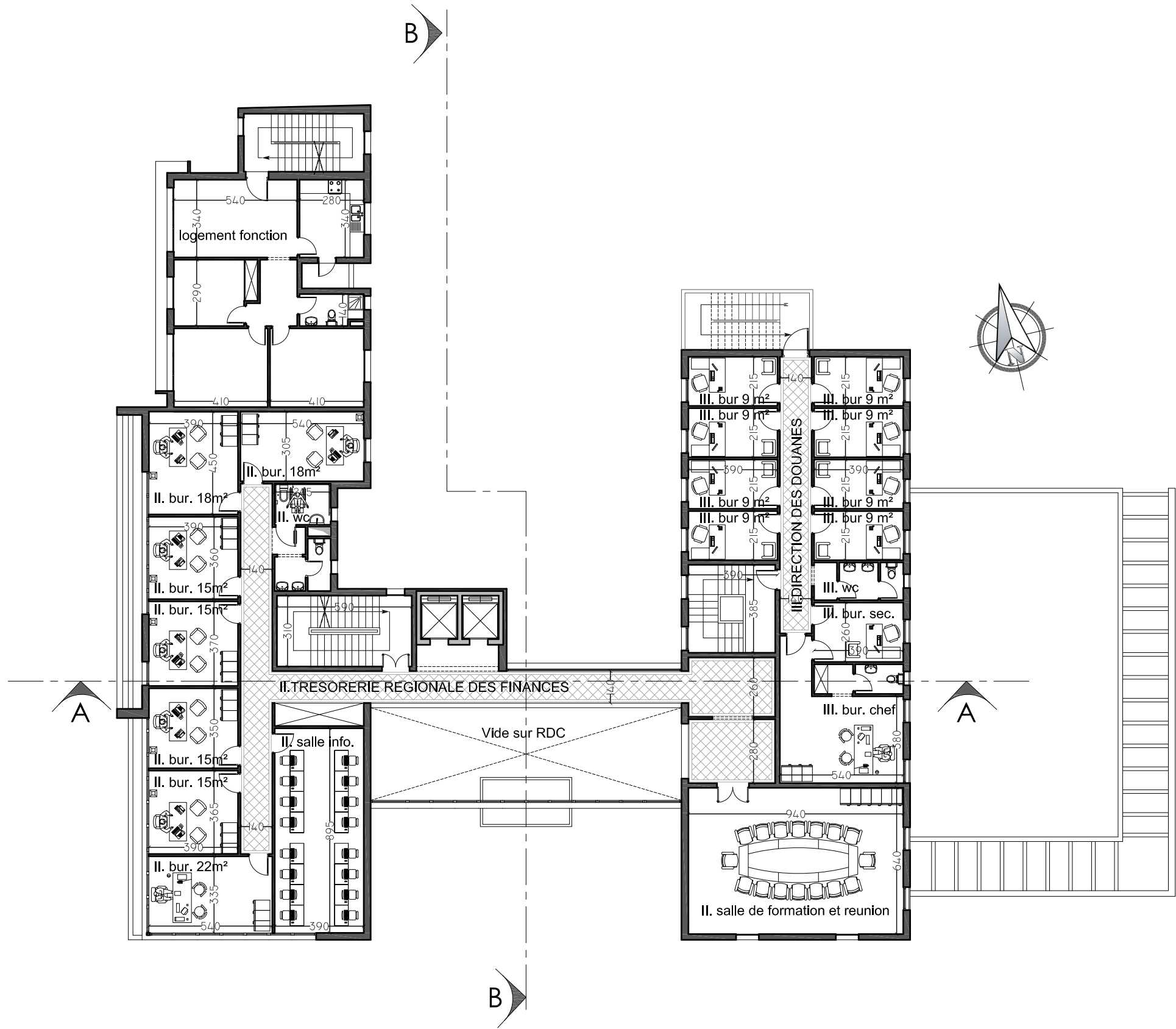
PLAN 2ème Etage ech 1/200
