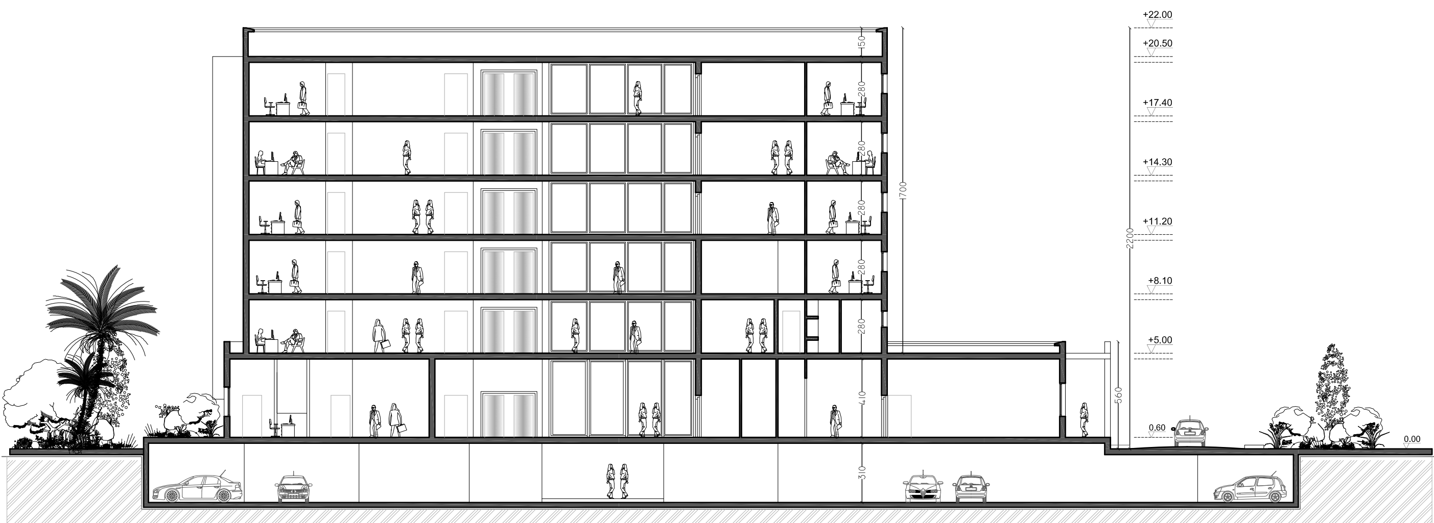
COUPE A-A ech 1/200
