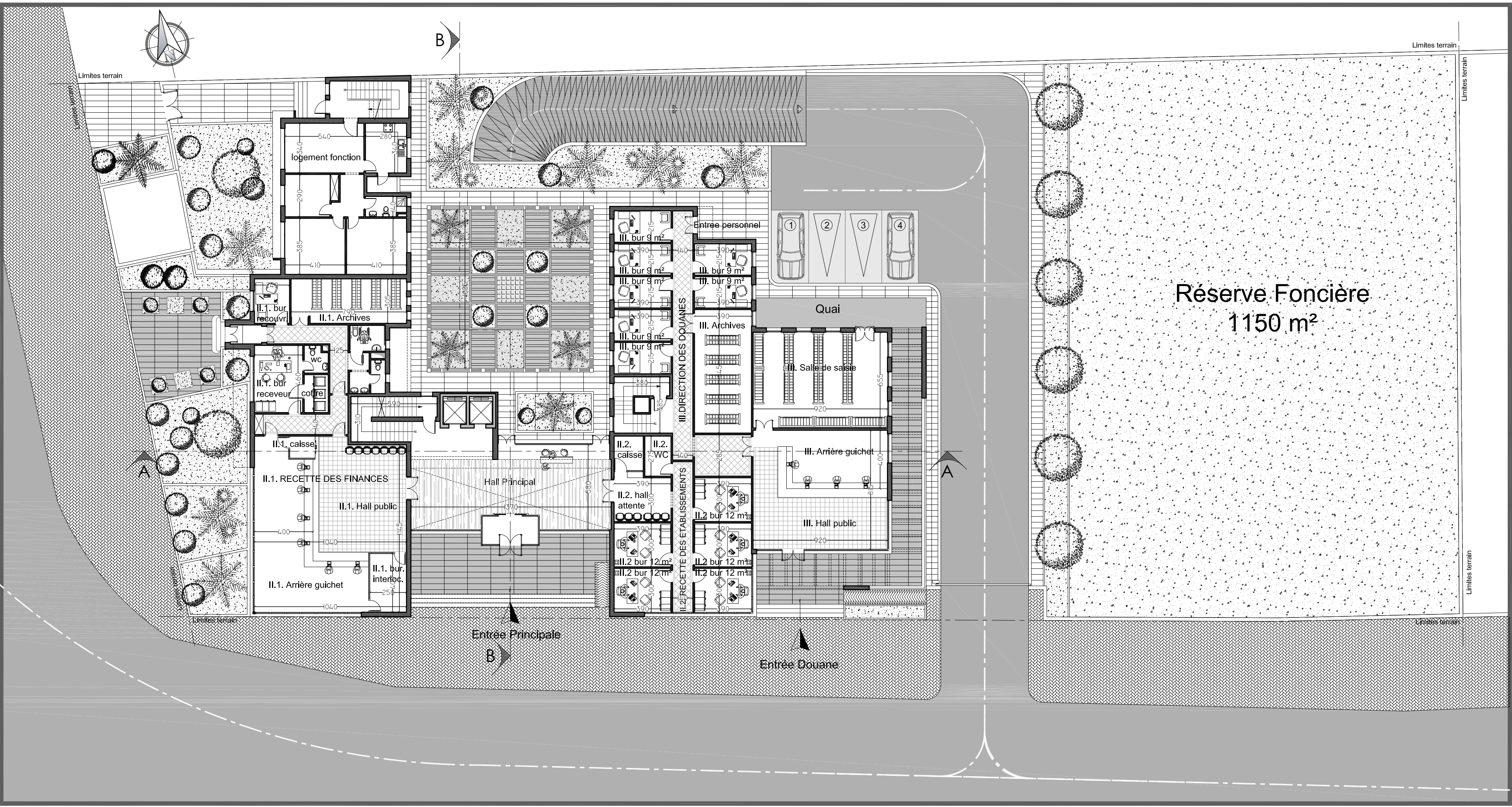
PLAN RDC ech 1/200
