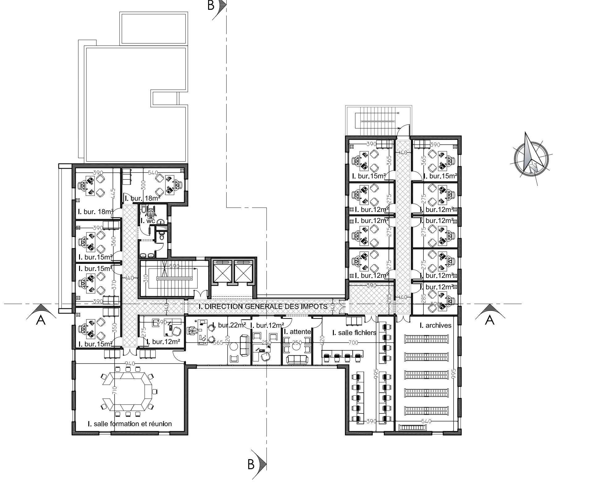
PLAN 4ème Etage ech 1/200
