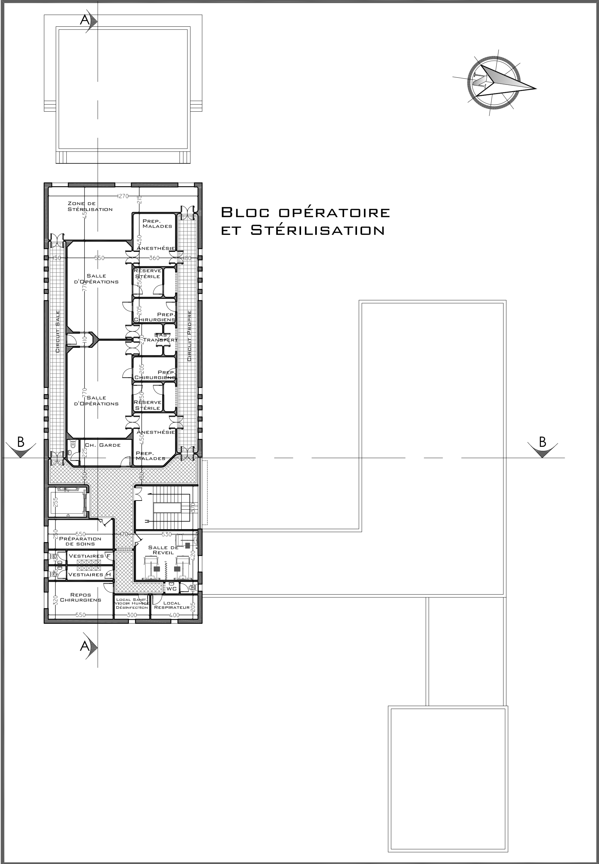
PLAN ETAGE ech 1/200
