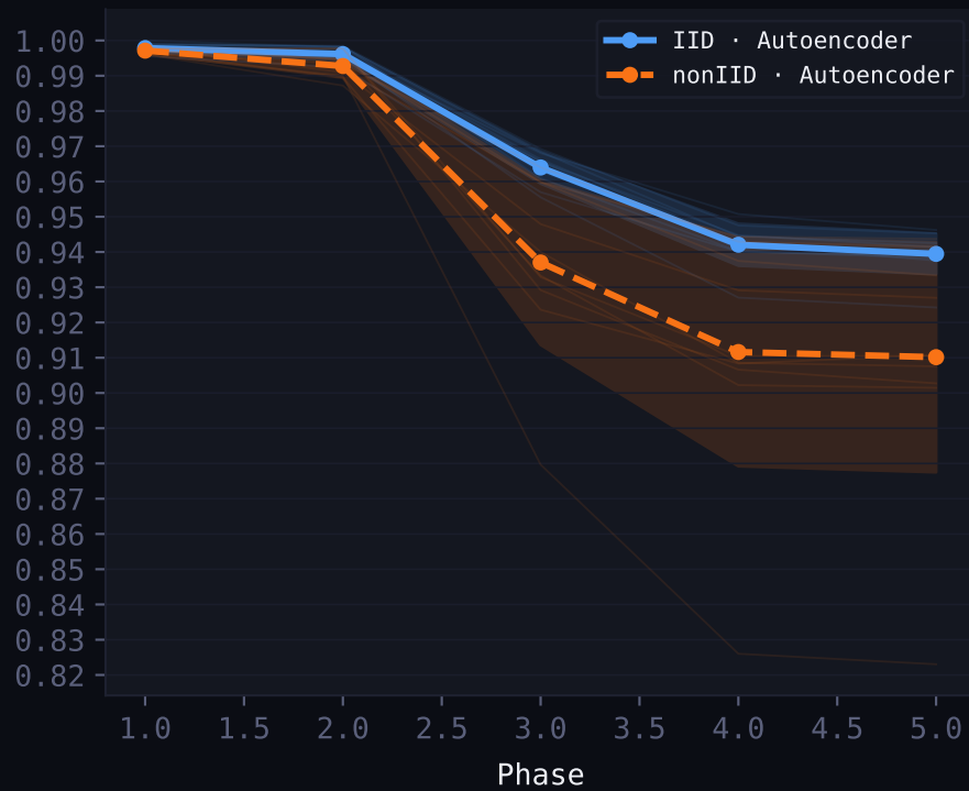
Autoencoder
