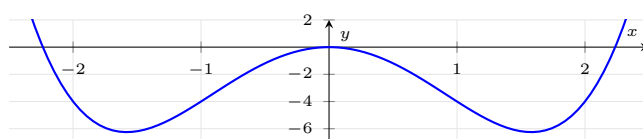
Soda funkcija y = x^4 - 5x^2
