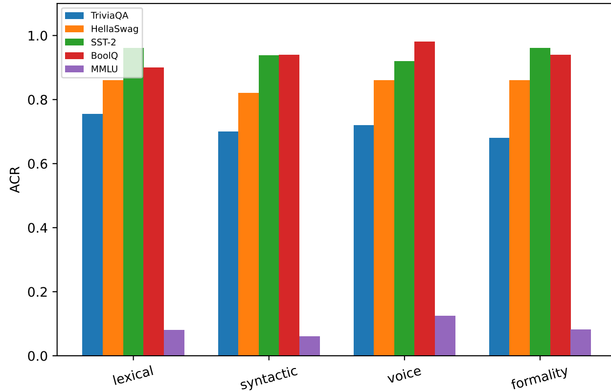
GPT-3.5-Turbo
