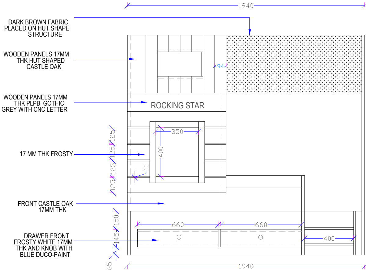
ELEVATION
