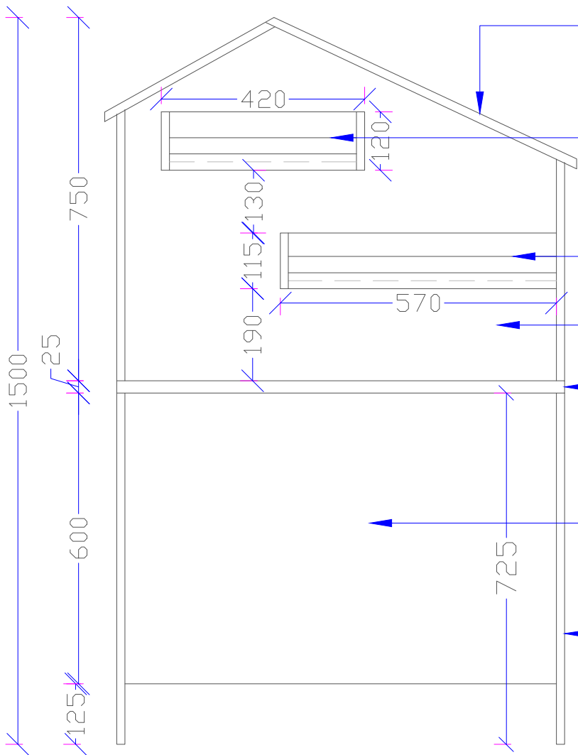
ELEVATION
