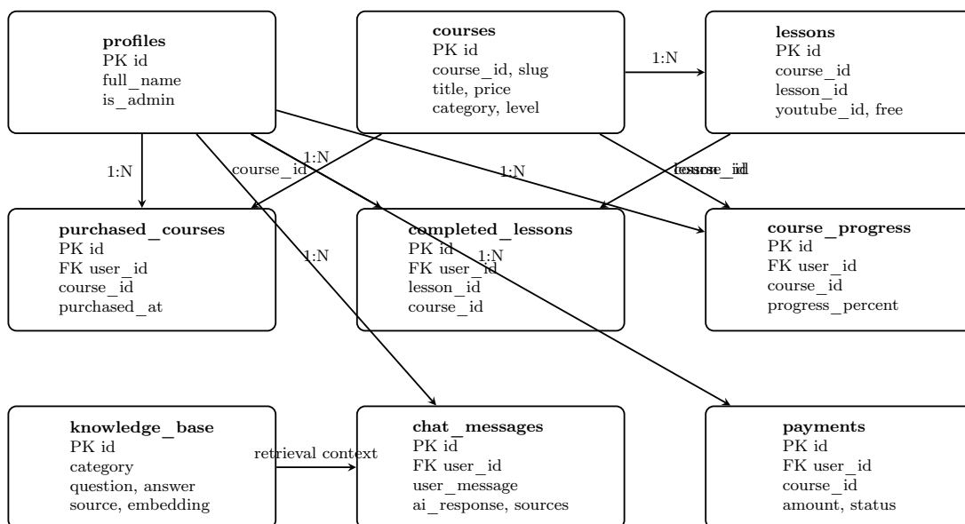
ЗУРАГ 4.5: Системийн үндсэн өгөгдлийн сангийн ER диаграм
