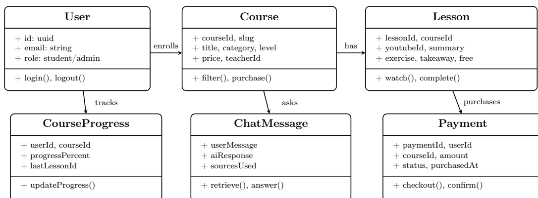
ЗУРАГ 4.4: Платформын домйин объектуудын класс диаграм
