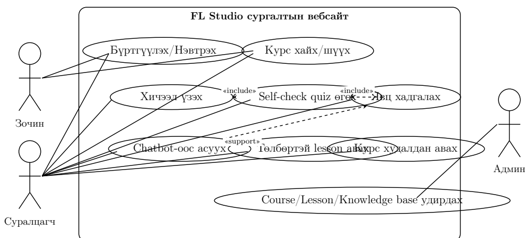
ЗУРАГ 4.2: FL Studio сургалтын платформын Use Case диаграм
