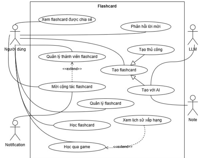
Hình 2.5: Use Case: Học tập với Flashcard
