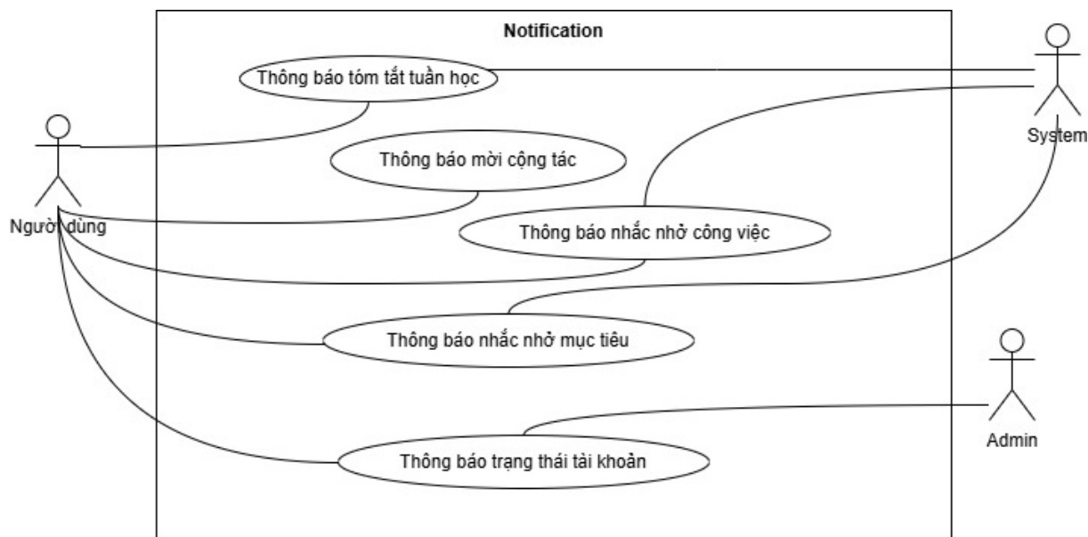
Hình 2.13: Use Case: Thông báo
