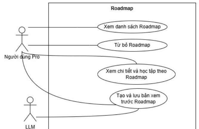
Hình 2.7: Use Case: Lộ trình học tập
