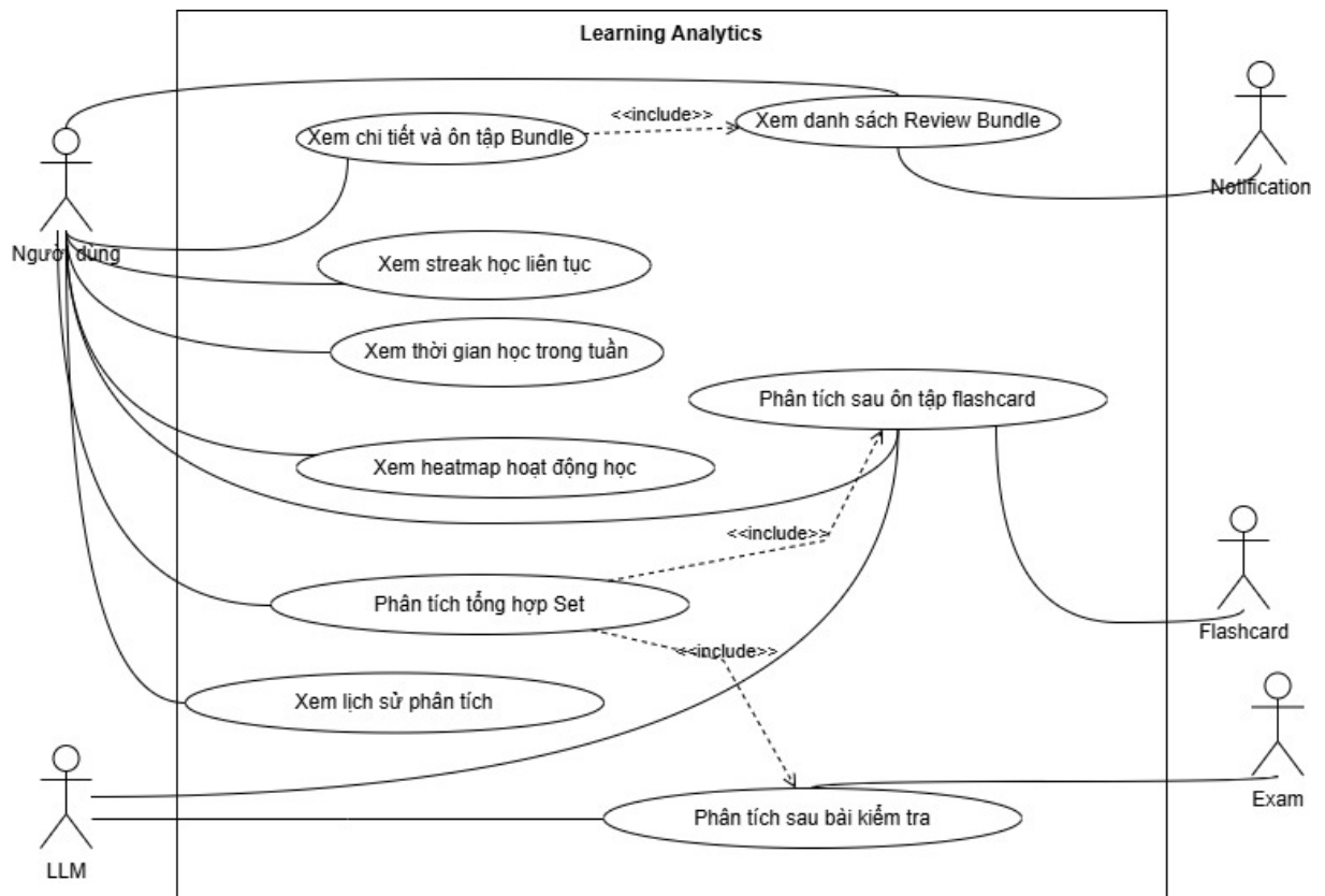
Hình 2.11: Use Case: Theo dõi và phân tích tiến trình học tập
