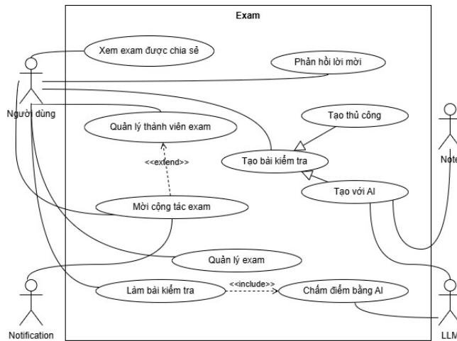
Hình 2.6: Use Case: Kiểm tra và đánh giá kiến thức
