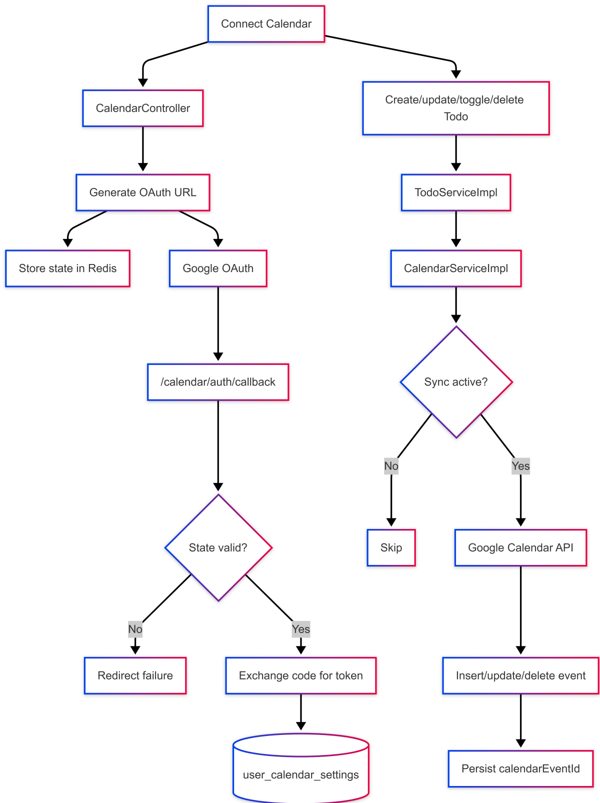
Hình 3.8: Luồng đồng bộ Todo với Google Calendar
