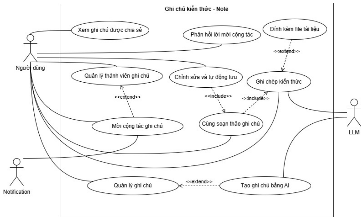
Hình 2.8: Use Case: Ghi chú kiến thức
