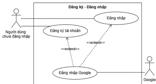
Hình 2.1: Use Case: Đăng ký và Đăng nhập
