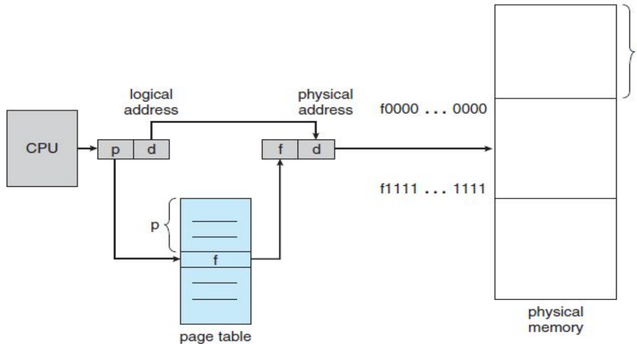
Figure 8.10 Paging hardware.
