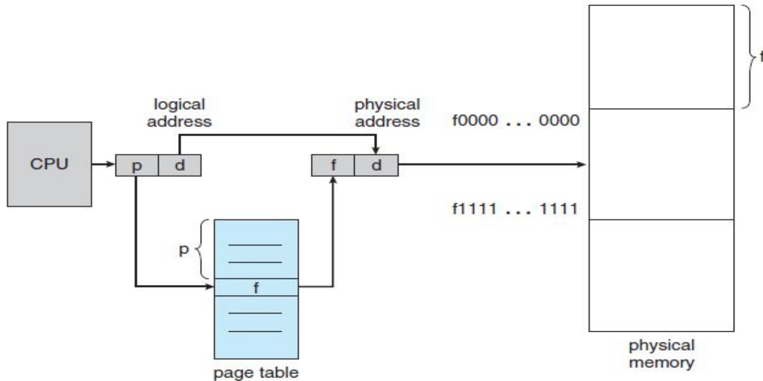
Figure 8.10 Paging hardware.
