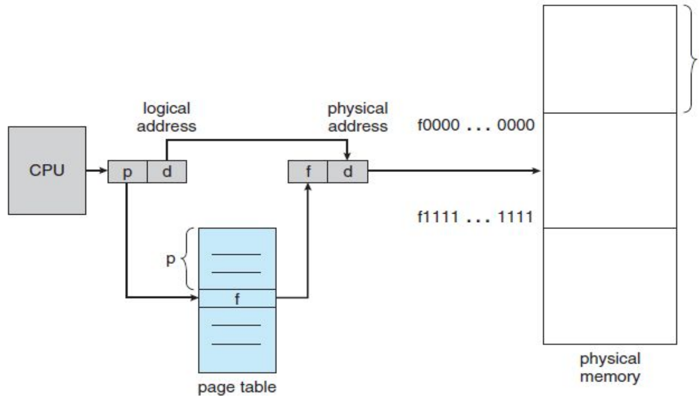
Figure 8.10 Paging hardware.
