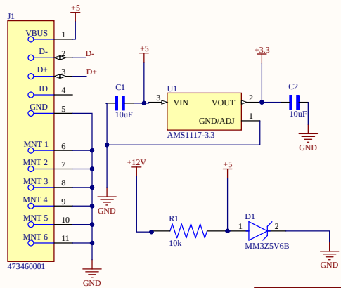
MICRO_USB
