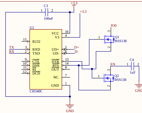
CH340C
