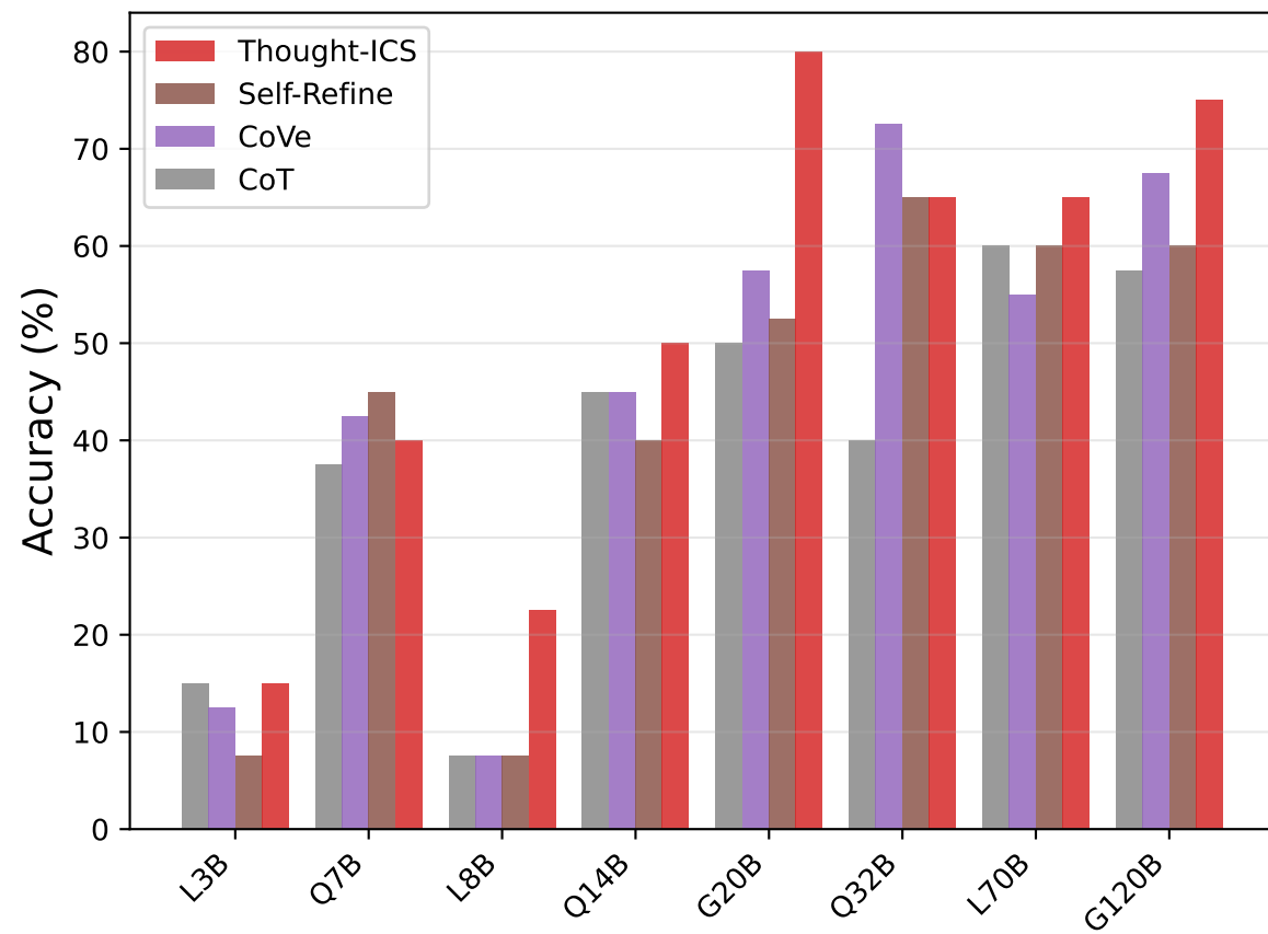
CSQA
