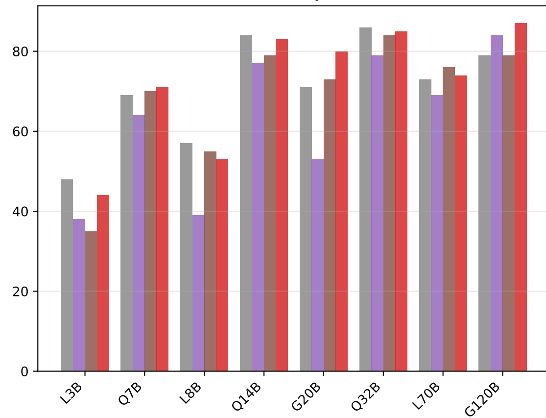
MathQA
