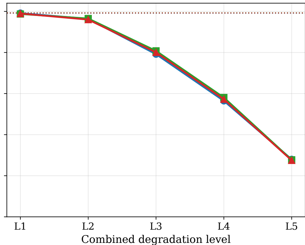
MNIST
