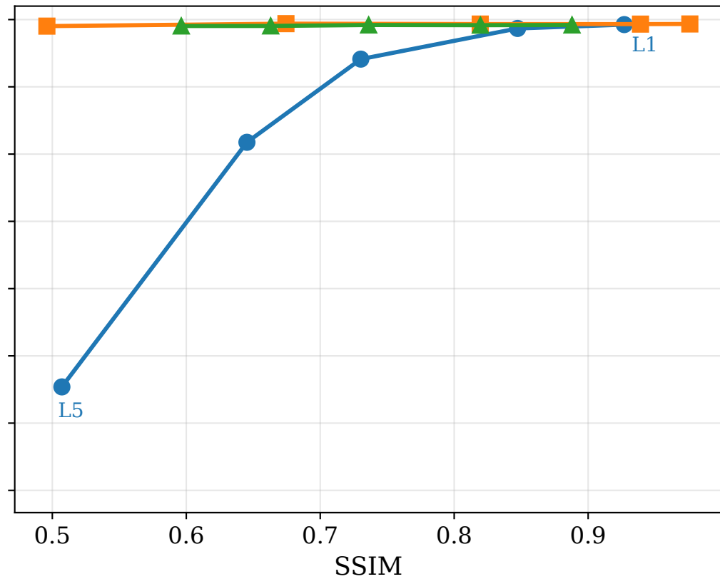
MNIST
