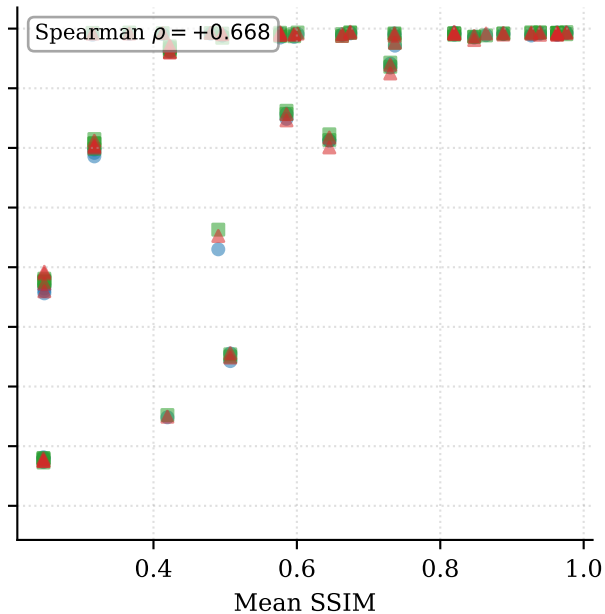
MNIST
