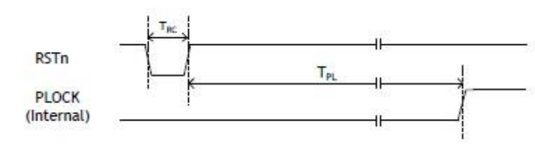
图 22 复位时钟
