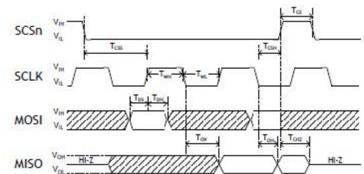
图 23 SPI 时钟
