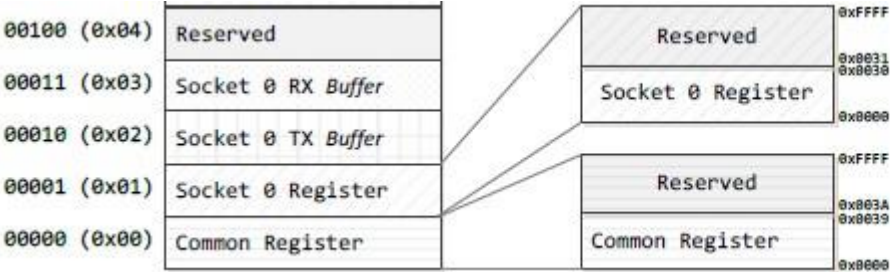
图 20 寄存器及内存构成
