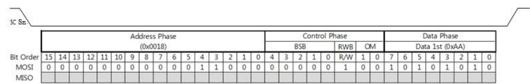
图 9 VDM 模式下，SIMR 寄存器写操作
