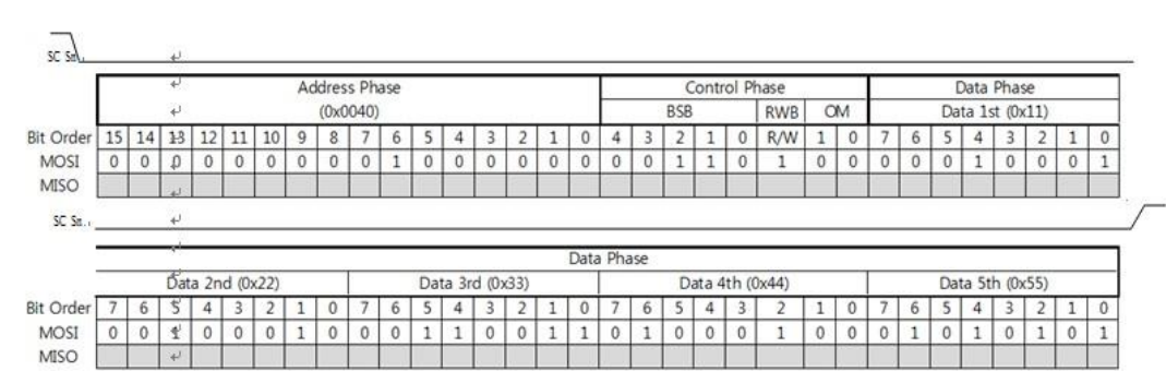
图 10 在 VDM 模式下，向 Socket1 的发送缓存区 0×0040 中写入 5 字节数据
