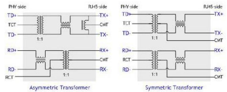
图 24 变压器类型
