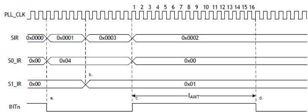
图 21 INTLEVEL 时序
