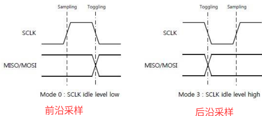
图 6 SPI 模式 0&3
