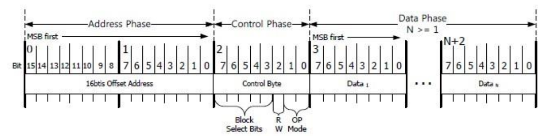
图 7 SPI 数据帧格式
